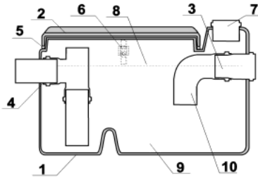
Принципова схема жируловлювача серії СЖ "Оптима"
