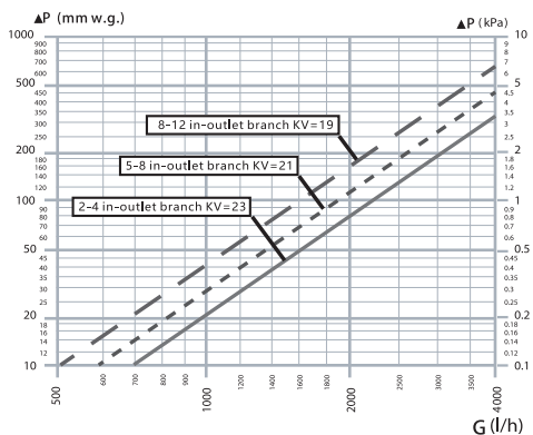
Рис. 2. Гидравлические характеристики
