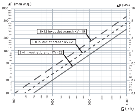
Рис. 2. Гідралічні характеристики
