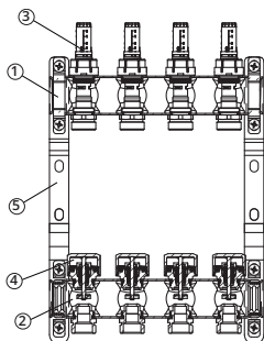
Таб. 1. Назначение элементов коллекторного блока
