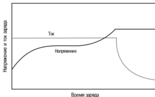
Рис. 2. График заряда при постоянном напряжении с ограничением начального тока заряда б) Заряд постоянным током (метод I)
