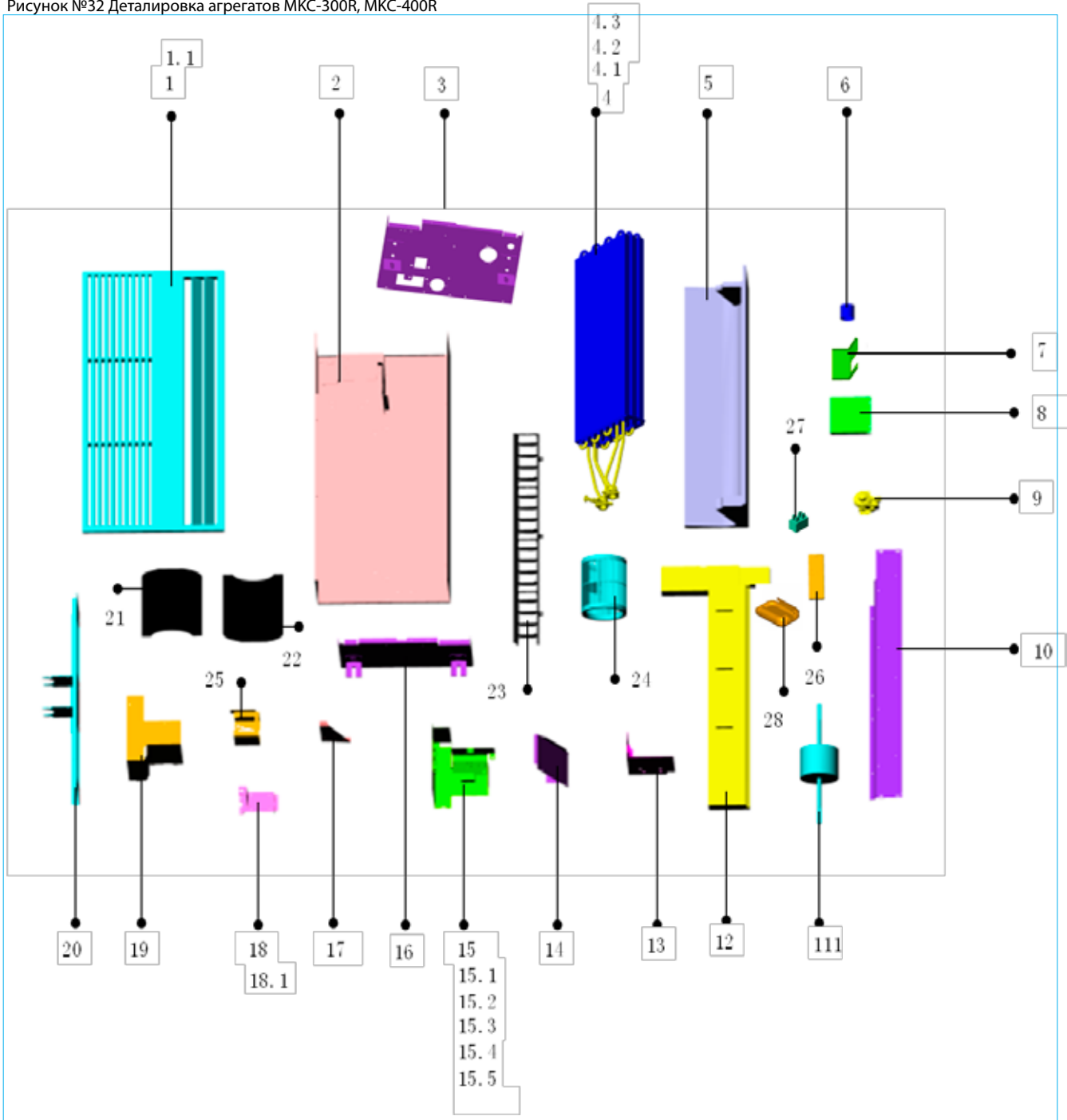
Рисунок №32 Детализовка агрегатов МКС-300R, МКС-400R
