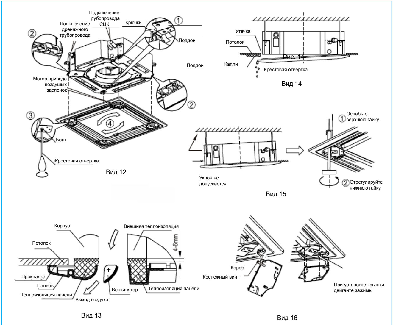
Рисунок №22 Монтаж панели
