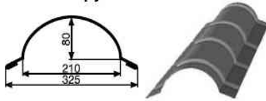
Рис. 8. Дахові аксесуари
