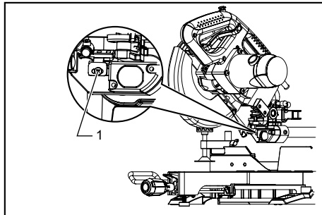
1. Laseryksikön kotelon ruuvi
