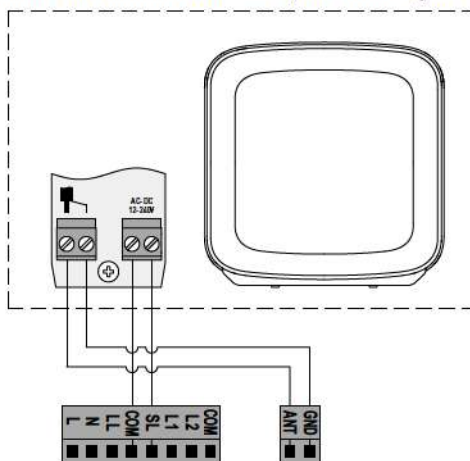
Рисунок 15. Схема подключения сигнальной лампы
