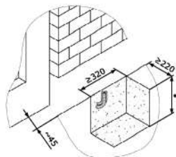
Рисунок 2. Подготовка под фундамент
