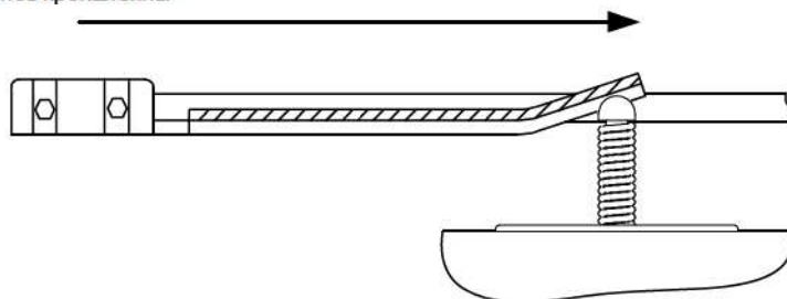
Рисунок 9. Кронштейн конечных положений
