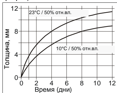
Граф. 1: Скорость отвердевания Sikaflex®-221
