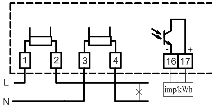
Рисунок 5.2 Схема підключення лічильника
