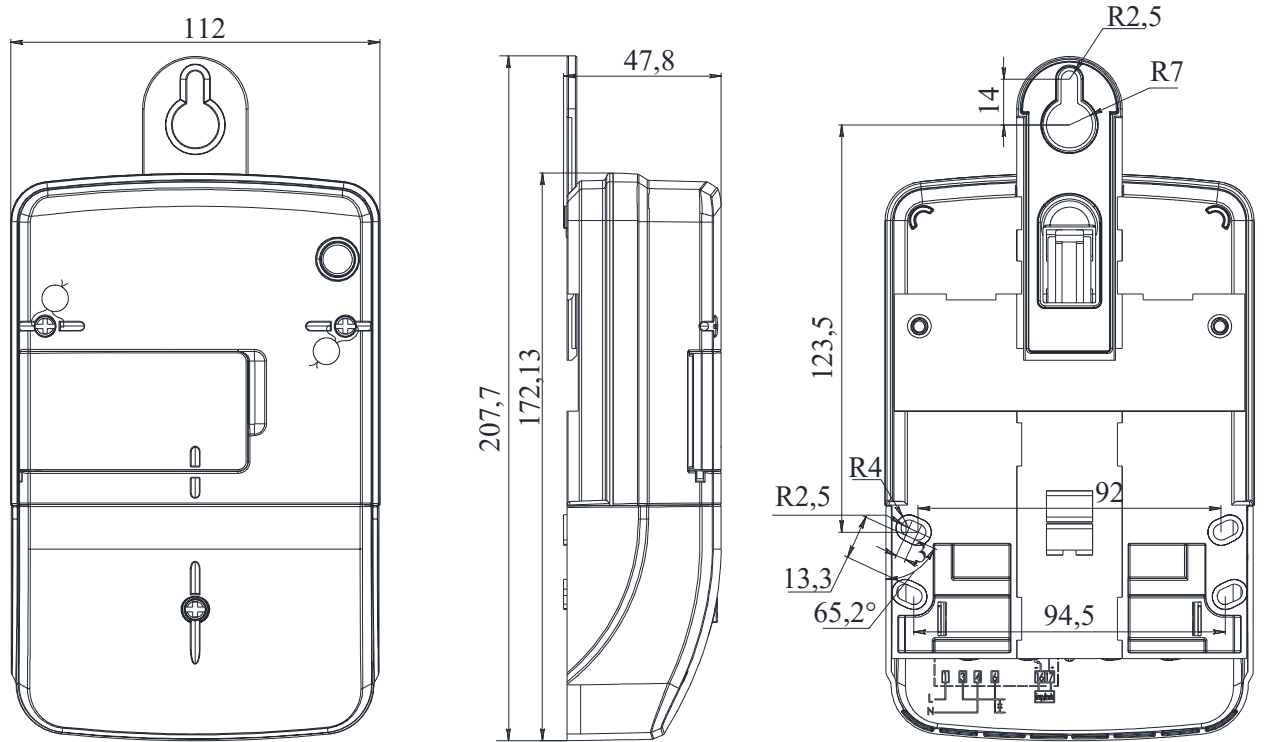
Рисунок 5.1 Габаритні та установчі розміри лічильника
