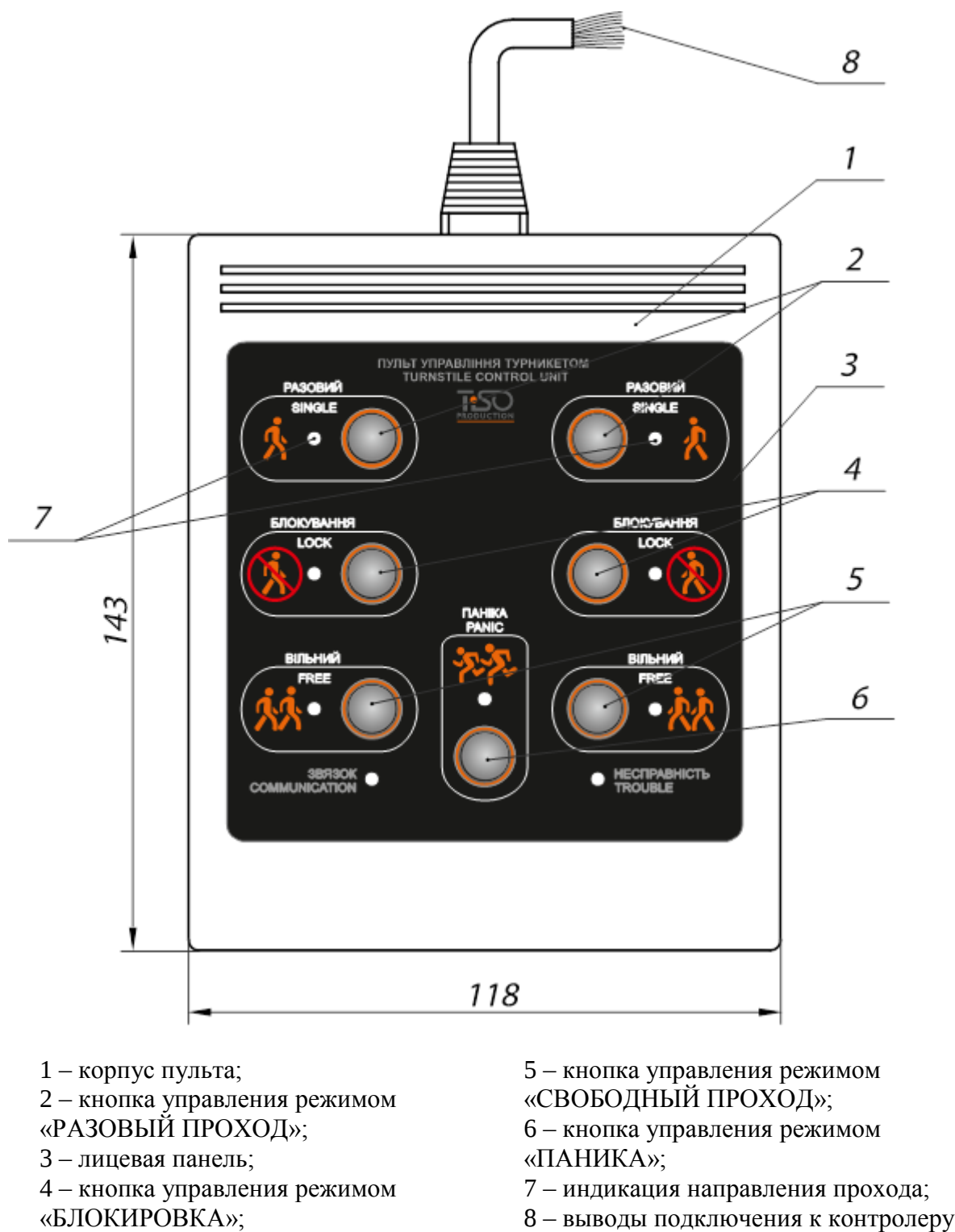
Рисунок Б.1 – Пульт управления АЮИА.114.02.00.00
