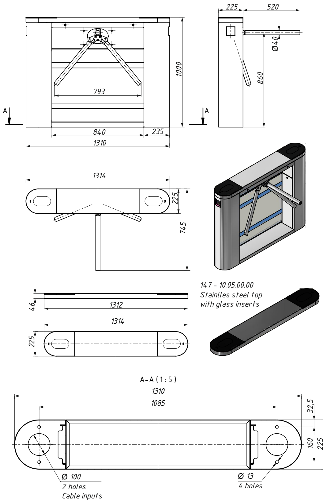
Рисунок А.1 – Турникет типа «трипод» GALAXY-M с крышкой из нержавеющей стали со стеклянной вставкой
