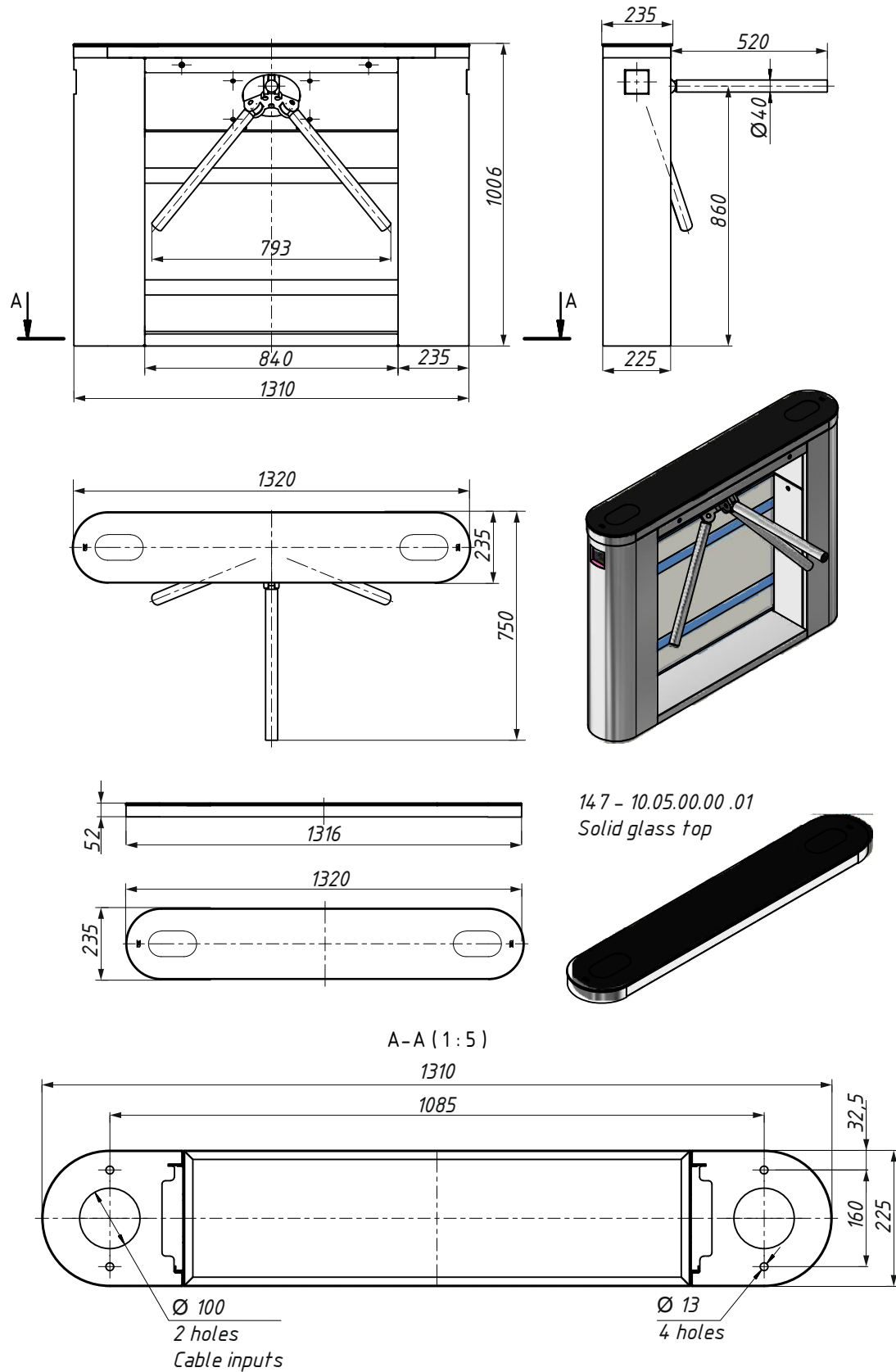
Рисунок А.2 – Турникет типа «трипод» GALAXY-M со сплошной стеклянной крышкой
