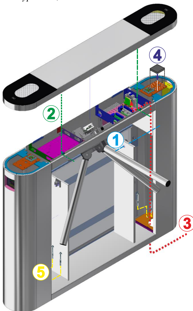
Рис. 16 – Общий вид сборки турникета-трипода «GALAXY-M»
