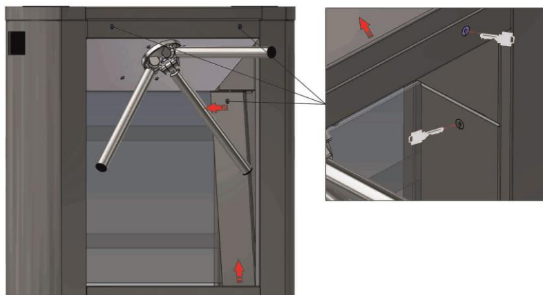
Рис. 15–Открытие двери и крышки турникета
