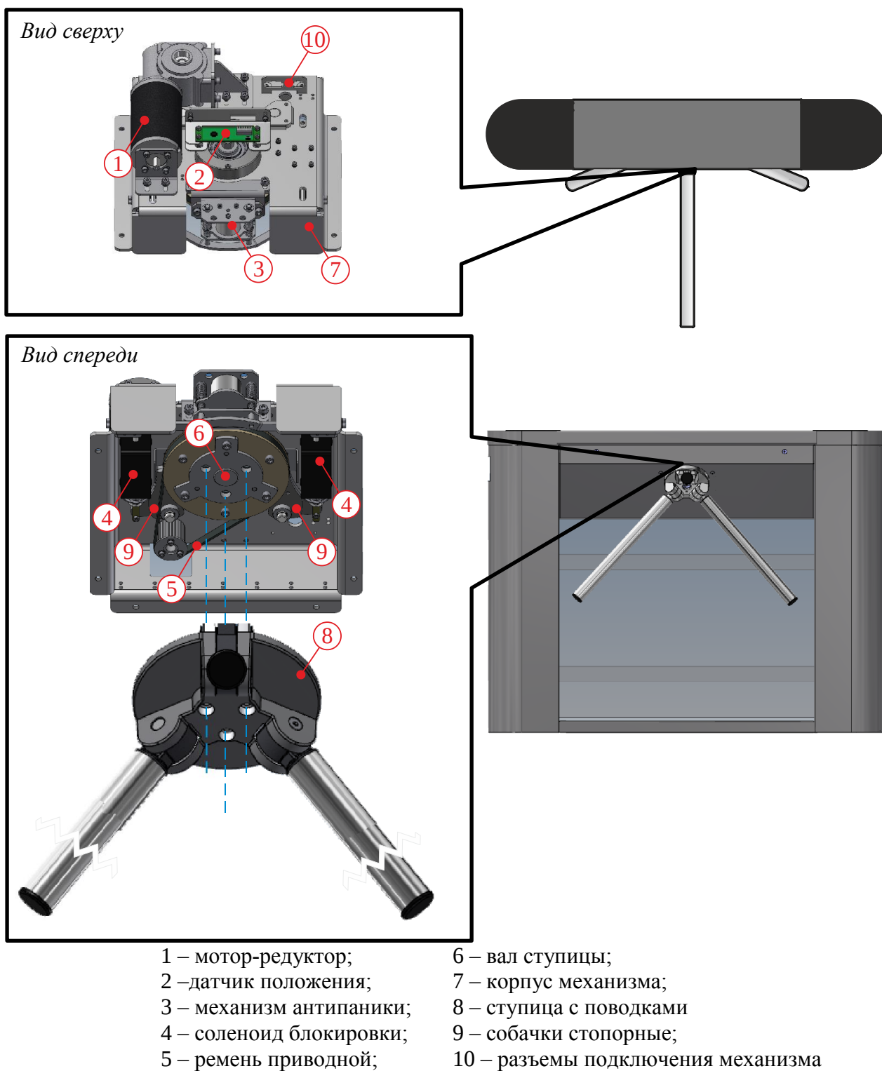
Рис. 5 – Рабочий механизм турникета
