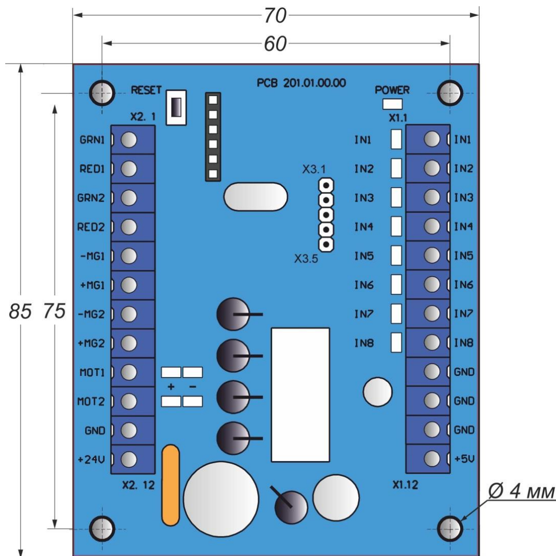
Рис. 9– Внешний вид контроллера моторизированного механизма PCB.201.01.00.00
