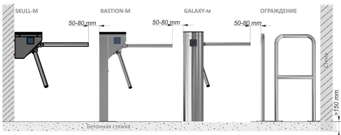
Рис. 11 – Варианты размещения турникетов (условно)
