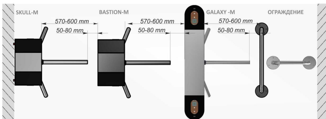
Рис.12 – Инсталляция размещения турникетов-триподов (условно)
