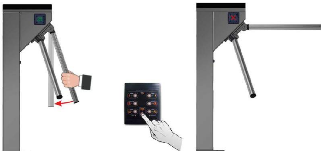
а) Положения поводка в режиме «ПАНИКА» перед восстановлением
