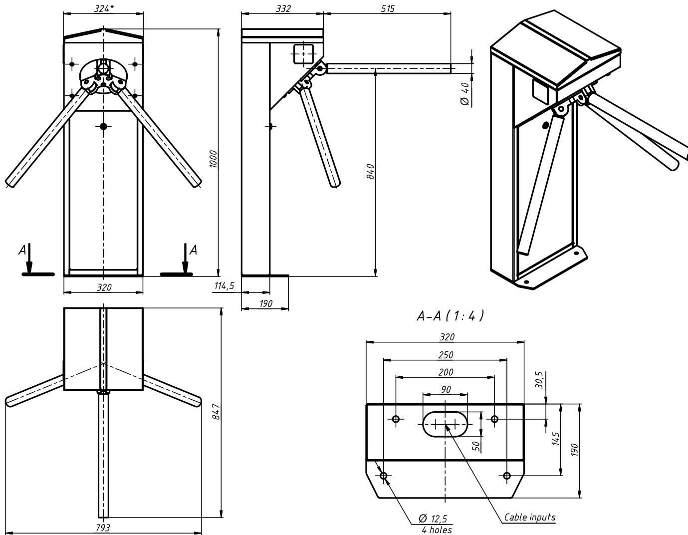
Рисунок А.1 – Турникет типа «трипод» CENTURION-M
