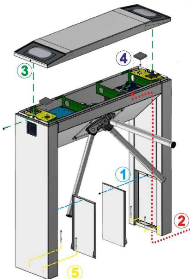
Рис. 16 – Общий вид сборки турникета трипода «TWIX-M»
