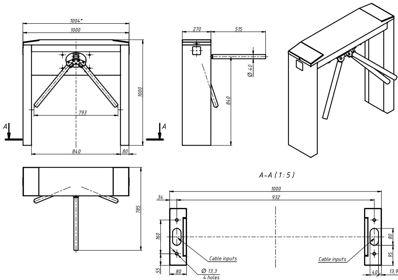
Рисунок А.4 – Турникет типа «трипод» TWIX-M
