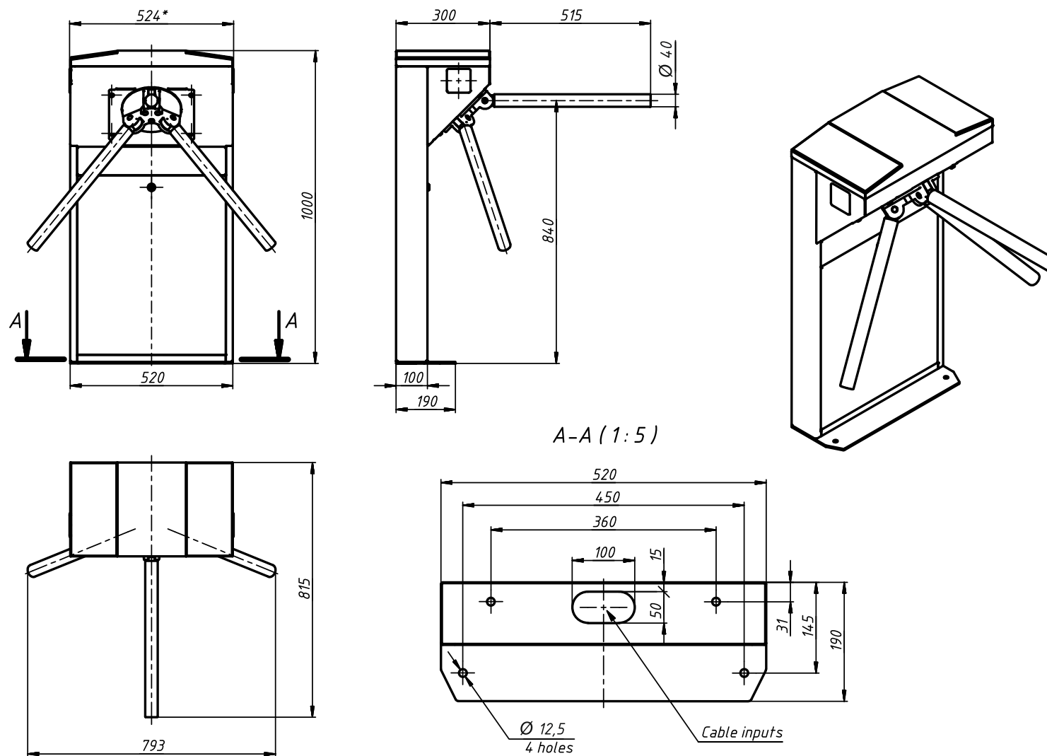
Рисунок А.2 – Турникет типа «трипод» BASTION-M
