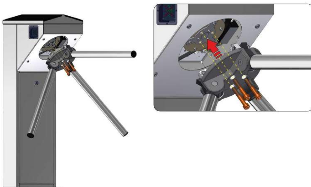
Рис. 14 – Установка ступицы с поводками в корпус турникета-трипода
