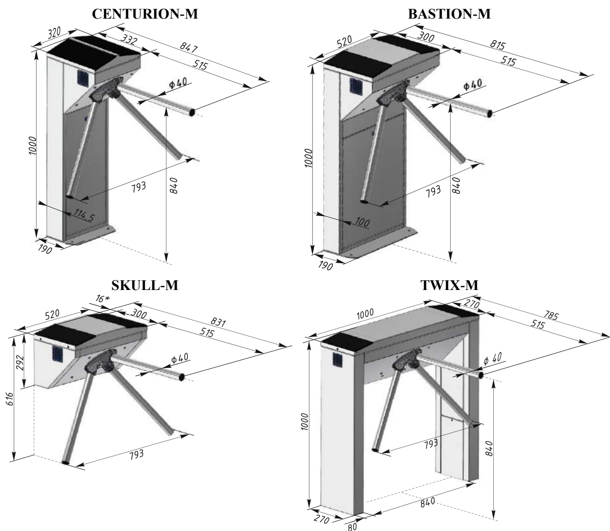
Рис. 3 - Габаритные размеры турникета-трипода
