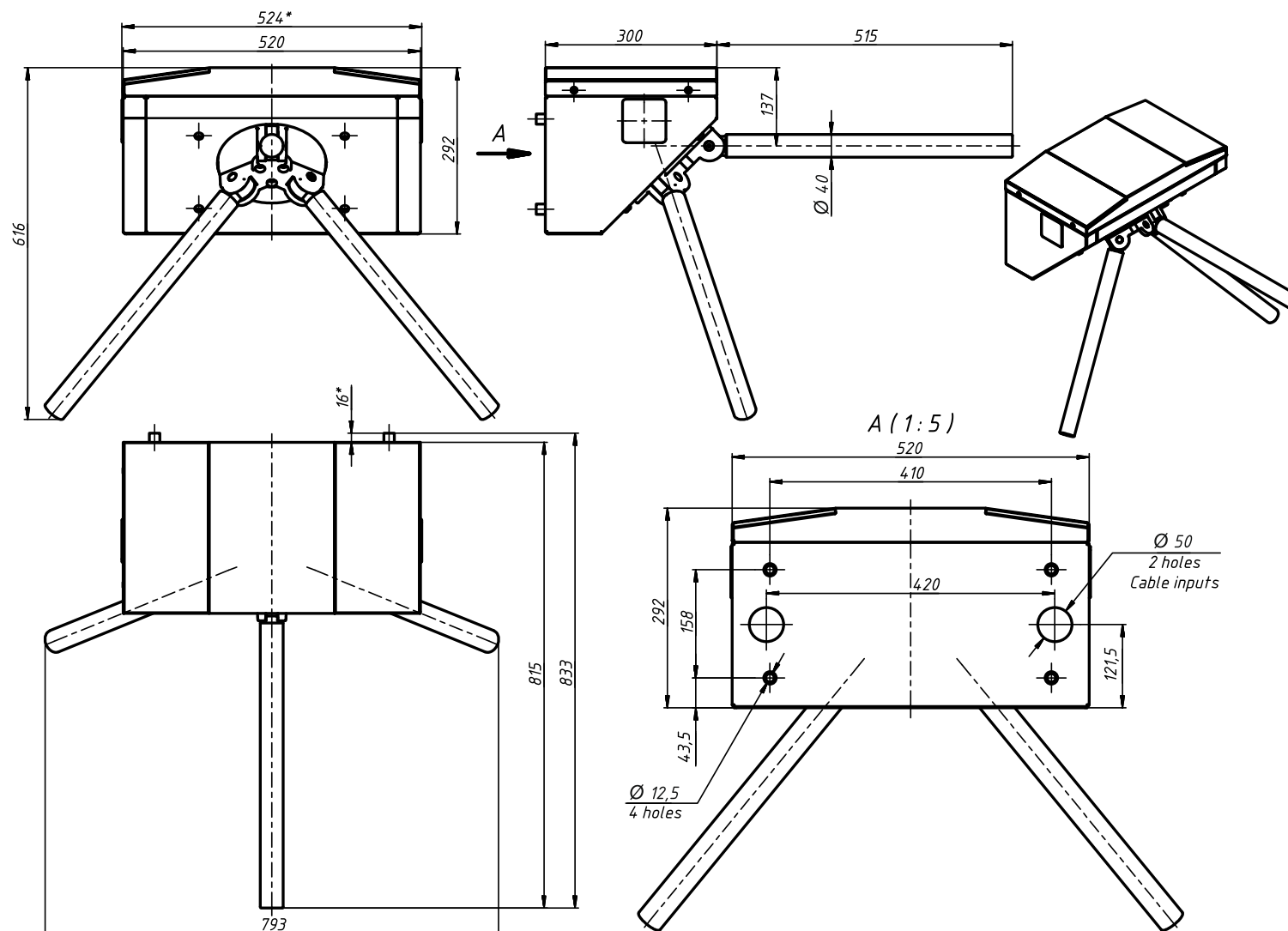
Рисунок А.3 – Турникет типа «трипод» SKULL-M
