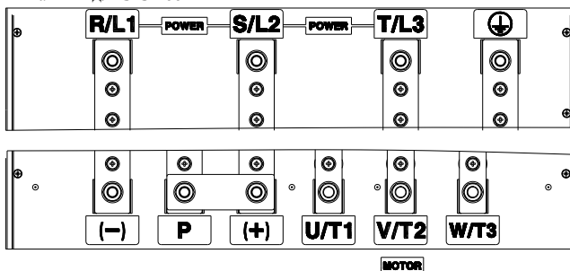
Рис.3-17 Схема выводов цепи питания 315~400 кВт
