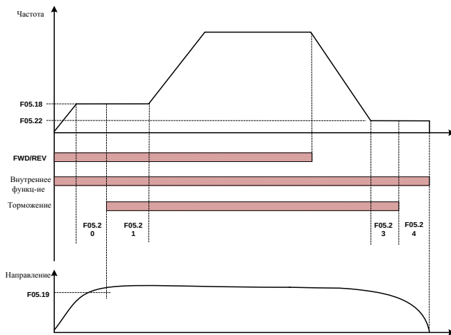
Fig 6-16 Логическая схема процесса управления торможением
