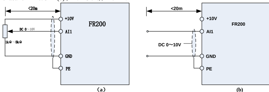
Рис. 3-20 Схема подключения вывода аналогового входа
