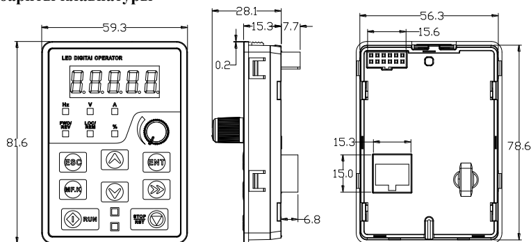
Рис. 2-10-а 0.75~2.2 кВт Габариты клавиатуры
