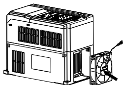
Рисунок 8-2 (а) Установка проводов вентилятора
