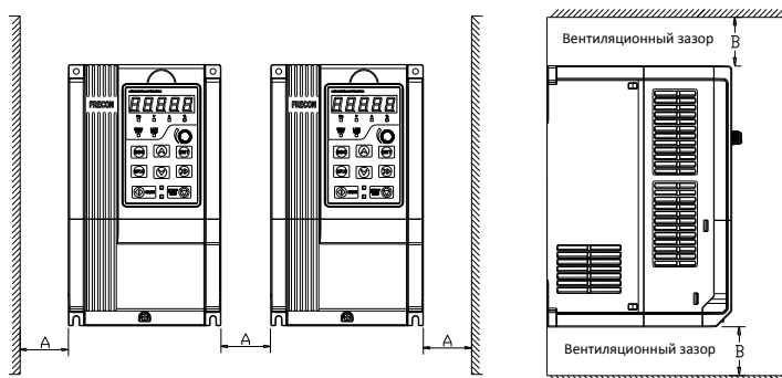
Рис.3-3 Ориентация при установке нескольких инверторов и требования к свободному пространству
