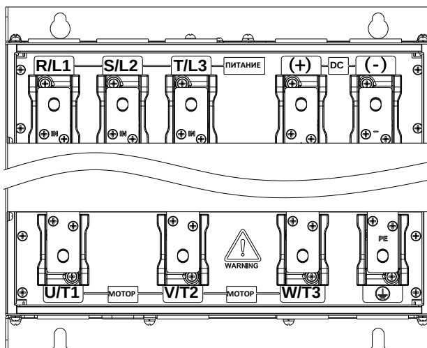
Рис. 3-16 Схема выводов цепи питания 90~280 кВт
