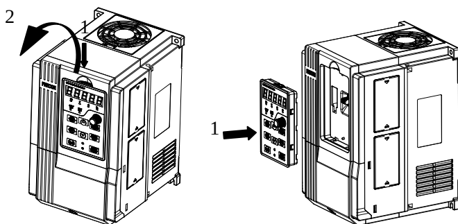
Рис.3-7(а) Удаление клавиатуры
