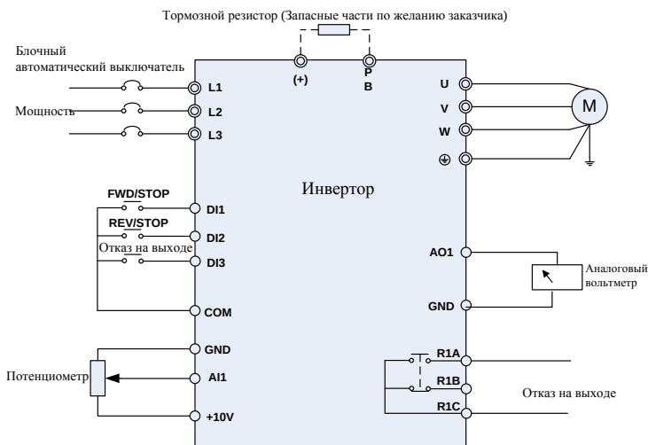
Рисунок 6 Объединенная схема
