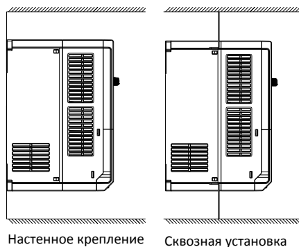
Рис.3-2 Ориентация при одиночной установке инвертора и требования к свободному пространству
