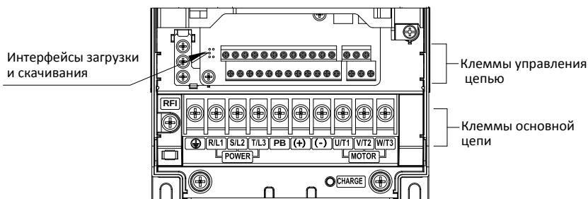
Рис. 3-12 Выводы цепи питания 4~15 кВт
