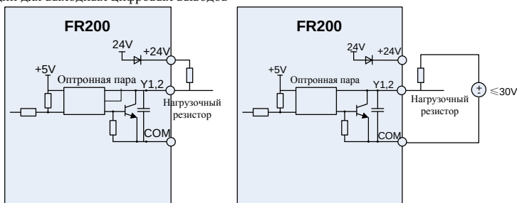
(а) Внутренний источник питания
