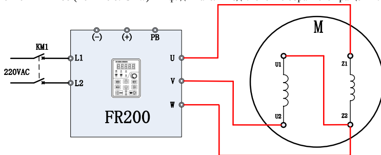
Рис. 6-19 Подключение ПЧ FR200 (меньше 0.75Kw) и 1-ф. двигателя подключение обратного вращения. (убрать конденсатор)
