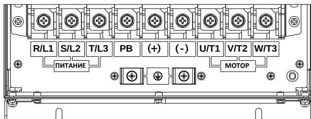
Рис. 3-15 Схема выводов цепи питания 37~75 кВт
