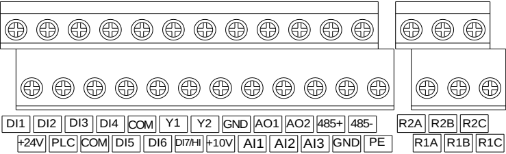
Рисунок 3 Схемы выводов управления серии FR200
