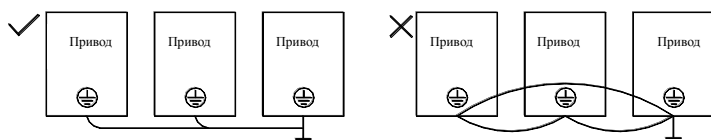
Рис. 3-28 Схема заземления инверторов
