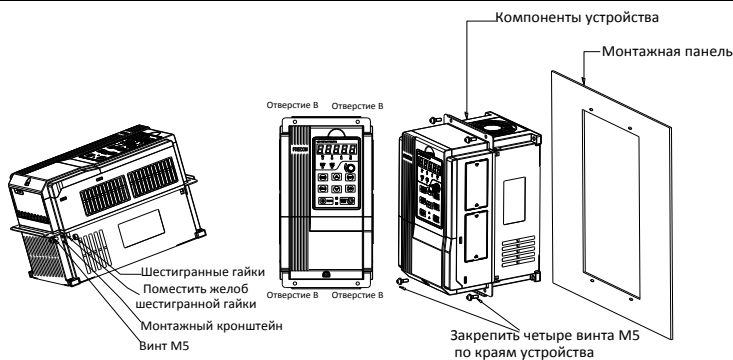
Рис. 3-6 (а) 0.75~15 кВт Настенный монтаж
