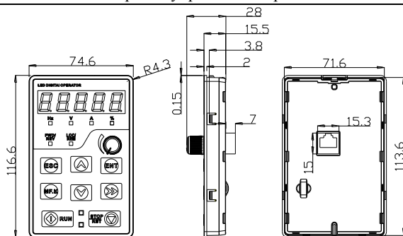
Рис.2-10-b 4.0~630 кВт Габариты клавиатуры
