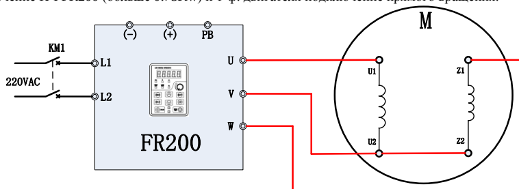
Рис. 6-20 Схема подключения ПЧ FR200 (больше 0.75KW) и 1-ф. двигателя подключение прямого вращения. (убрать конденсатор)
