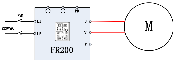
Рис. 6-23Схема подключения ПЧ FR200 (больше 0.75KW) и 1-ф. двигателя (не убирать конденсатор)
