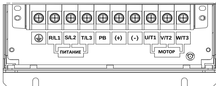
Рис. 3-13 Схема выводов цепи питания 18.5~30 кВт
