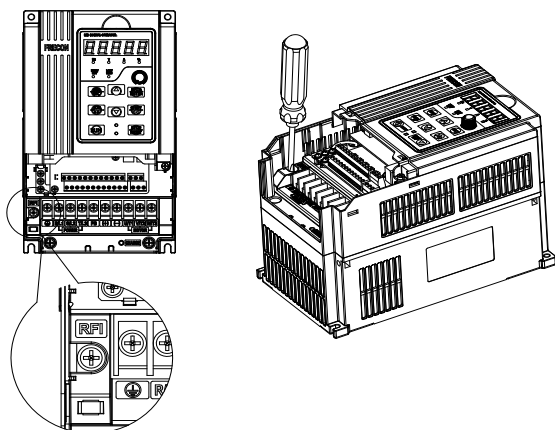
Рис. 3-26 4.0~15кВт схема перемычки RFI
