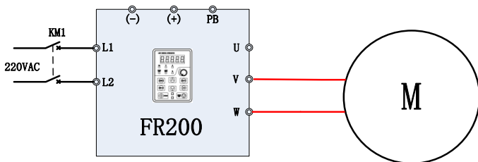
Рис. 6-22 Схема подключения ПЧ FR200 и 1-ф. Двигателя (не убирать конденсатор)
