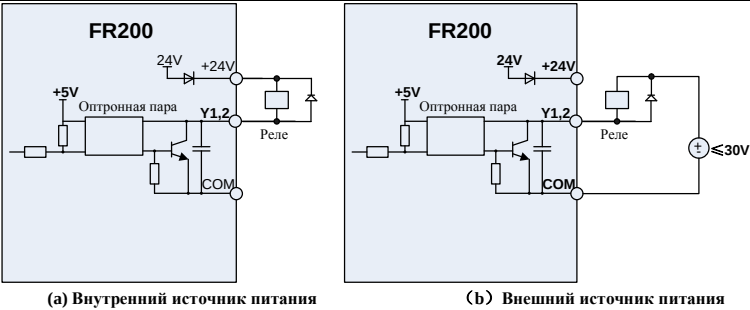
Рис. 3-25 Схема подключения, когда Y2 и НО – реле привода
