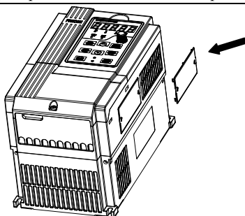
Рис. 3-8 Установка и удаление пылезащитной крышки
