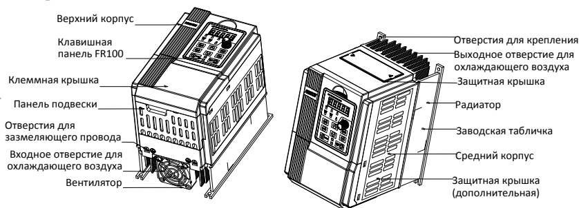
Рис. 2-3-а 3 Пример компоновки 0.75 ~ 2.2 кВт
