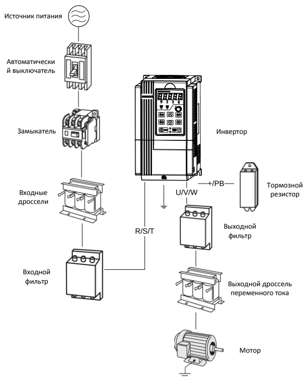
Рис. 3-9 Стандартная конфигурация периферийных устройств
