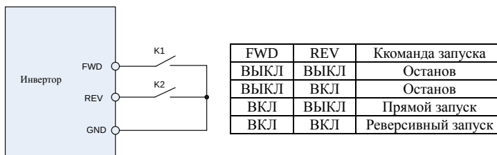
Рисунок 6-9 Установка двухпроводного режима 2
