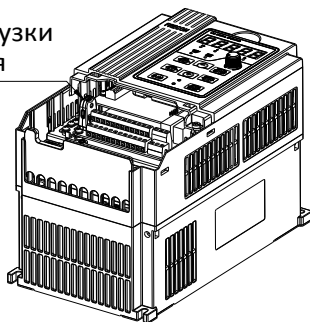
Рисунок В-2 Установка модуля передачи и скачивания
