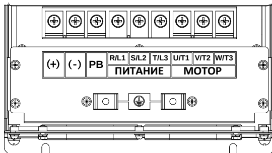
Рис. 3-13 Схема выводов цепи питания 18.5~30 кВт
