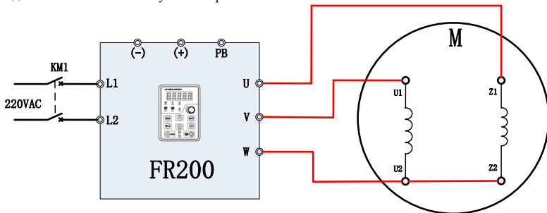
Рис. 6-18 Схема соединительного провода FR200 (меньше 0.75KW) и однофазного двигателя прямого вращения (убрать конденсатор)
