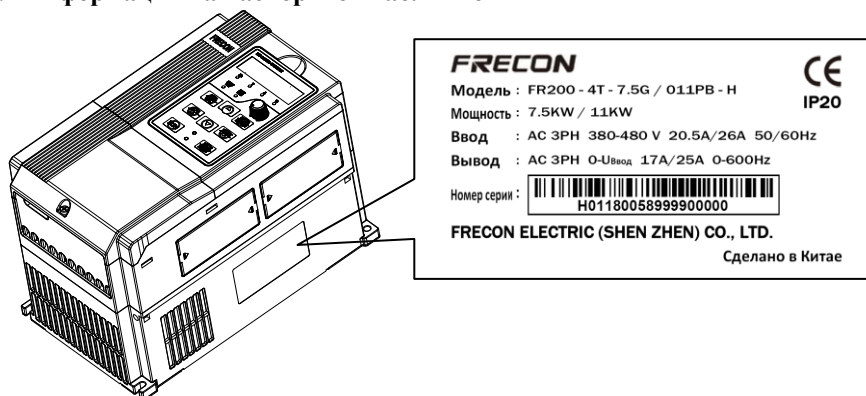
Рис. 2-1 Информация на паспортной табличке
