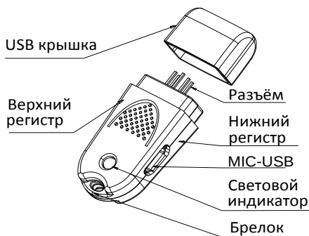
Рисунок В-1 Внешний вид модуля загрузки и скачивания
