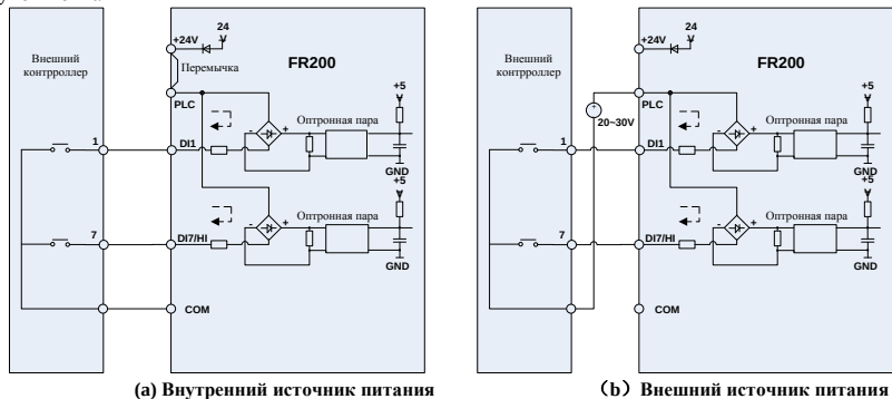
Рис. 3-21 Сухой контакт
