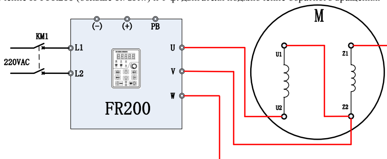
Рис. 6-21 Схема подключения ПЧ FR200 (больше 0.75KW) и 1-ф. двигателя подключение обратного вращения. (убрать конденсатор)
