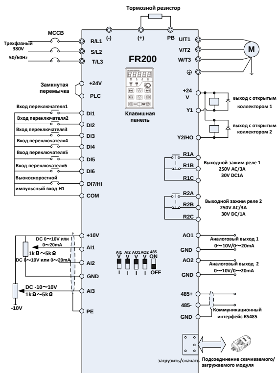
Рис. 3-10 Монтажная схема инвертора FR200
