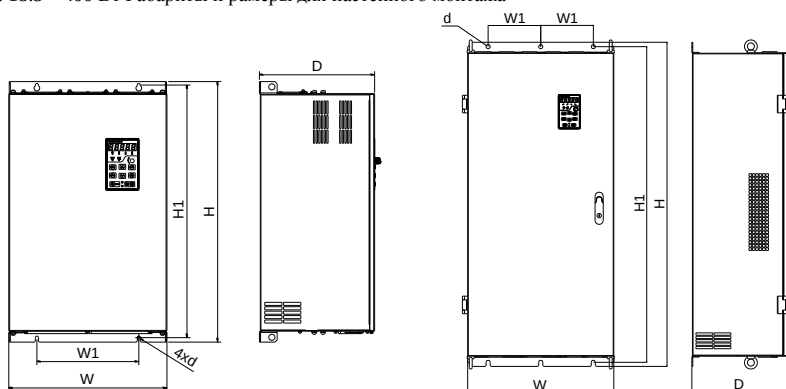
Рис. 2-6 18.5~132 кВт Схема настенного монтажа (1) 160~400 кВт Схема настенного монтажа (2)
