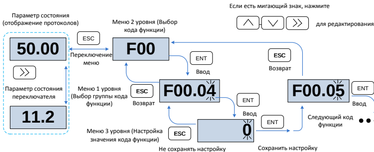
Рис.4-2 Рабочие процедуры при использовании клавиатуры
