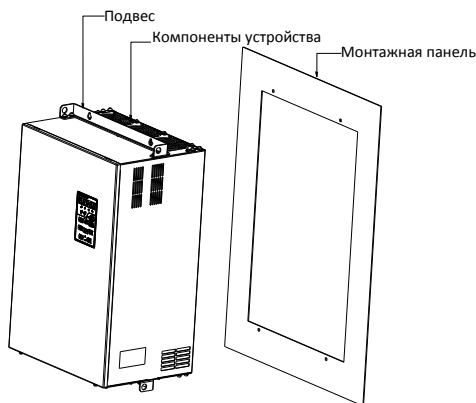
Рис. 3-6 (b) 18.5~132 кВт Настенный монтаж
