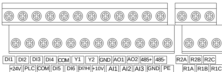
Рис. 3-19 Клеммы цепи управления
