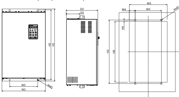
Рис. 2-9 18.5~132 кВт Схема установки на монтажном фланце
