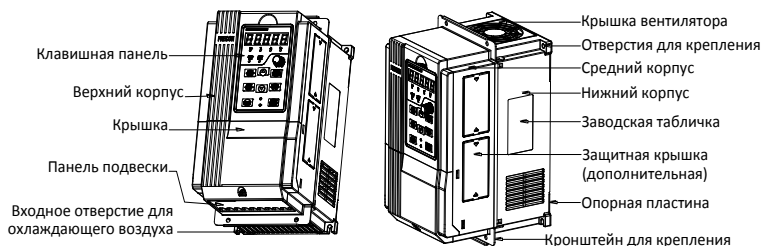
Рис. 2-3-б 3 Пример компоновки 4 ~ 15 кВт
