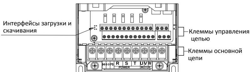
Рис. 3-11 Выводы цепи питания 0.75~2.2 кВт
