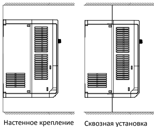
Рис. 3-1 Методы установки
