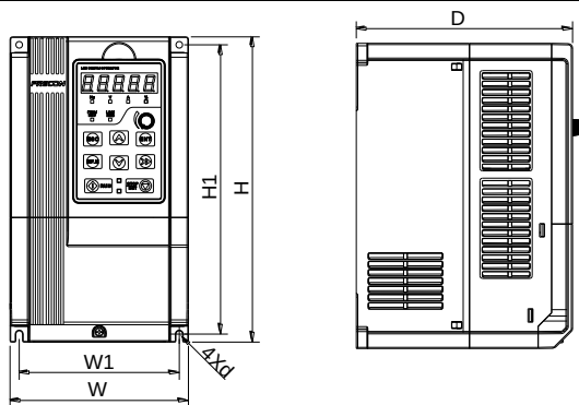
Рис. 2-5 0.75~15 кВт Схема настенного монтажа
