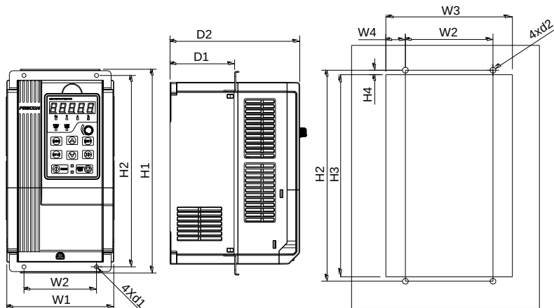
Рис. 2-8 0.75~15 кВт Схема установки на монтажном фланце
