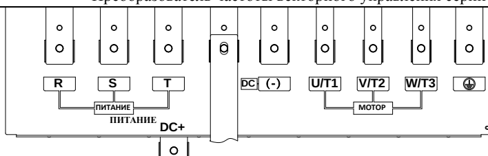
Рис.3-18 Схема выводов цепи питания 450~630 кВт
