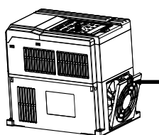
Рисунок 8-2 (b) Установка крышки вентилятора
