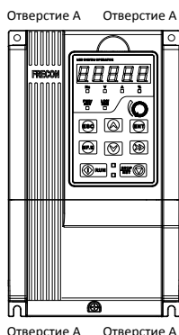
Рис.3-5 Настенный монтаж
