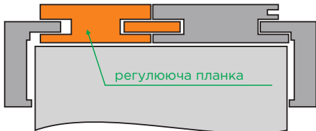
Переріз дверної коробки із регулюючою планкою та шпонкою
