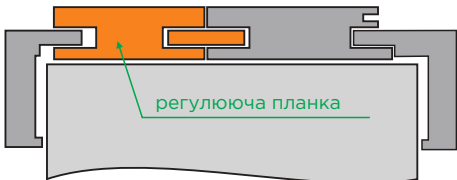
Переріз дверної коробки із регулюючою планкою та шпонкою
