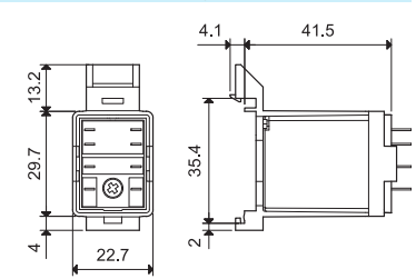
056.27 с реле
