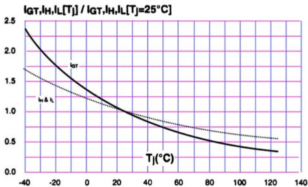
7、门极触发特性曲线
