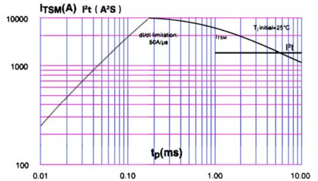
6、 I_{TSM}-t, I_{pt}-t 曲线
