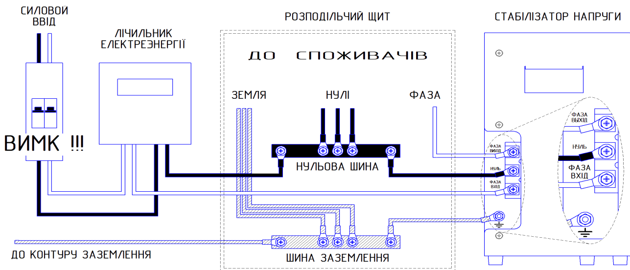
Малюнок 2. Рекомендована схема підключення стабілізатора до мережі.
