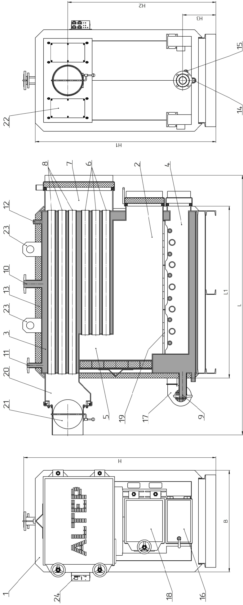
Рисунок 1 – Зовнішній вигляд та основні елементи котла
