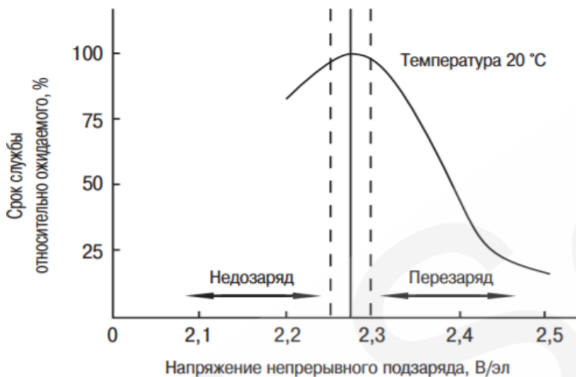
Рис. 13 Зависимость срока службы аккумулятора от напряжения подзаряда.
