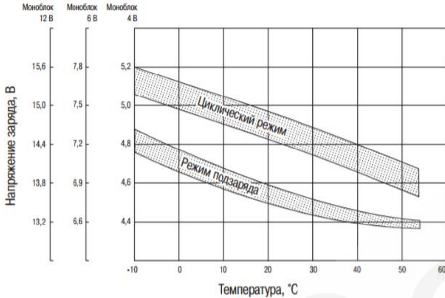
Рис. 10 Соотношение между напряжением заряда и температурой.
