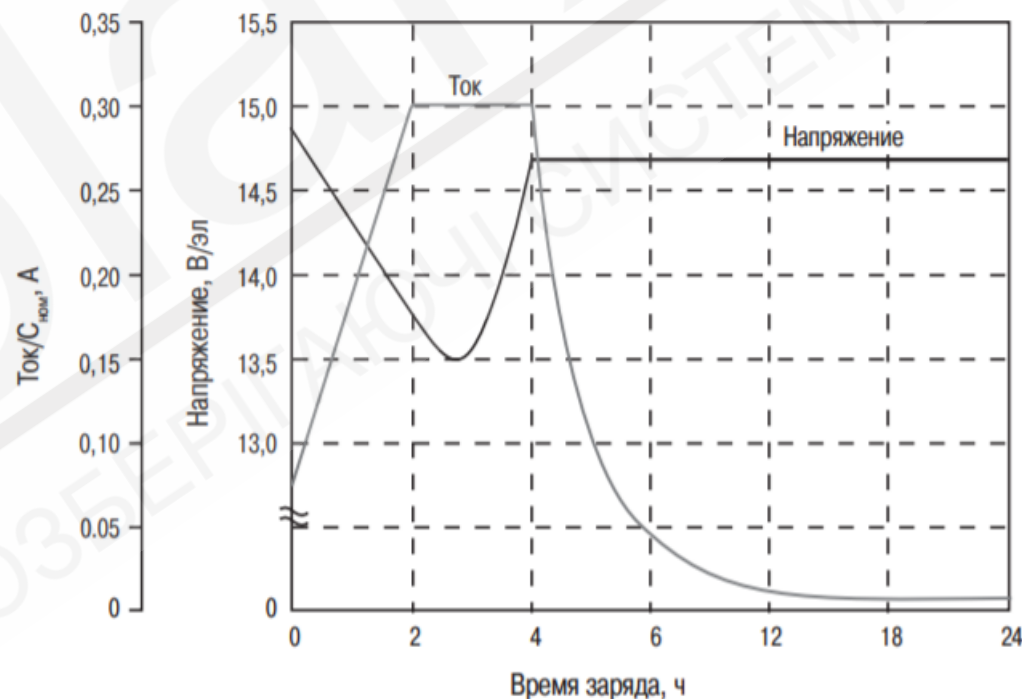
Рис. 7 Зарядные характеристики после глубокого разряда.
