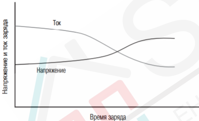
Рис. 5 График заряда падающим током.
