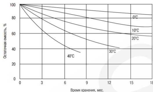
Рис. 1 Характеристики саморазряда аккумулятора.
