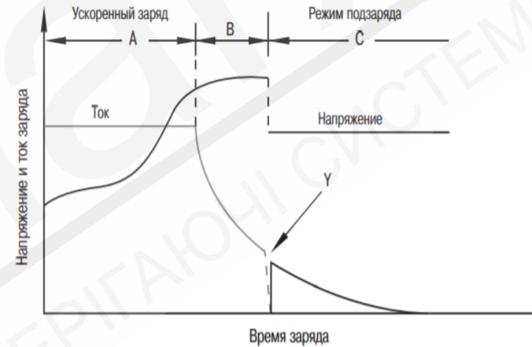
Рис. 6 Зарядные характеристики при использовании двухступенчатого заряда постоянным напряжением.
