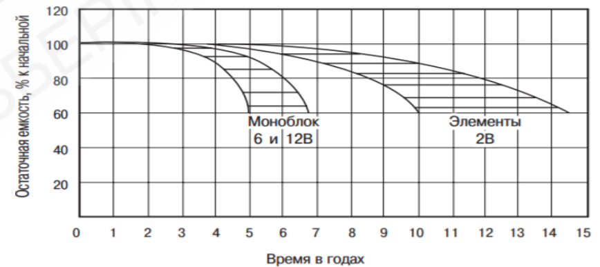
Рис. 12 Срок службы аккумулятора, работающего в режиме постоянного подзаряда.
