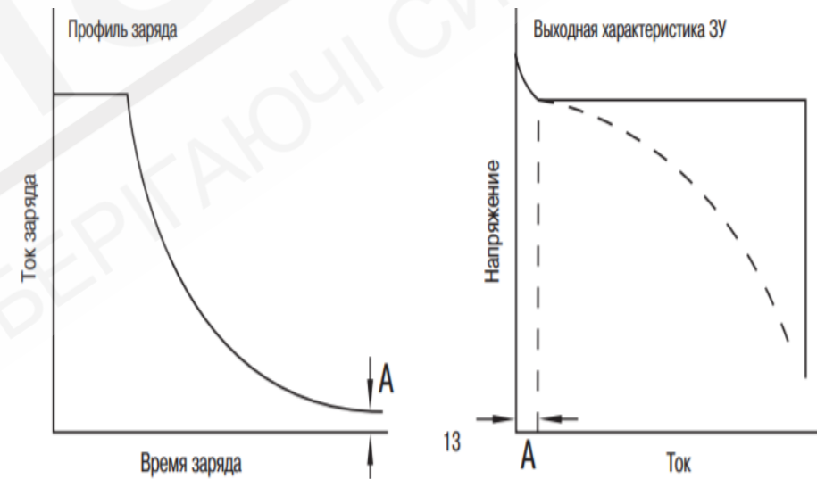
Рис. 8 Зарядная характеристика и выходная характеристика зарядного устройства.
