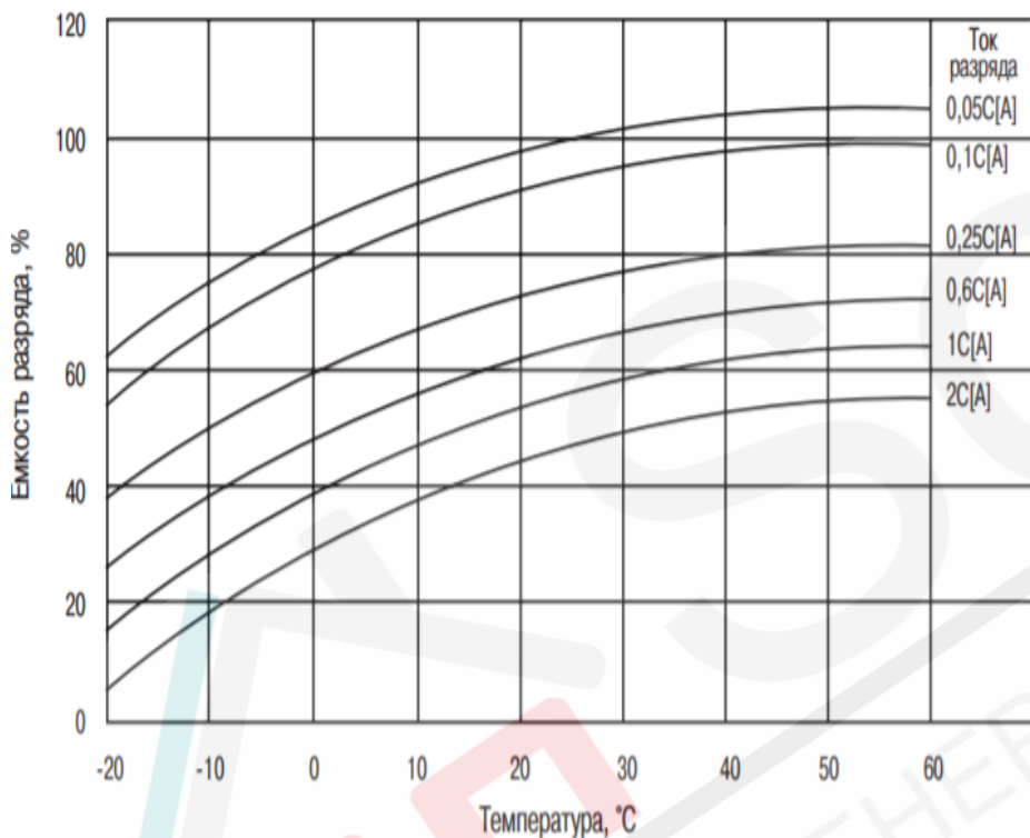
Рис. 9 Влияние температуры на емкость аккумулятора.
