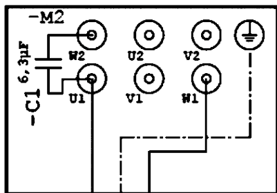
Схема подключения
