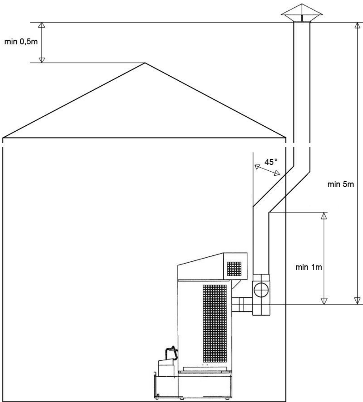
Рис. 3 Дымоходная система
