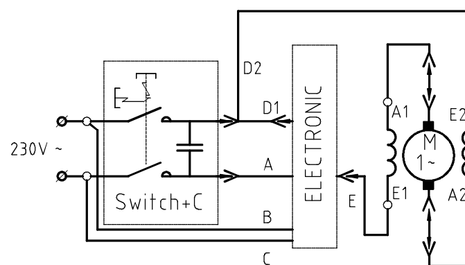
СХЕМИ НА СВЪРЗВАНЕ
