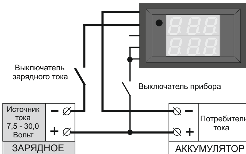
Рис. 5. Вариант измерения зарядного тока и напряжения на аккумуляторе и измерения уровня заряда аккумулятора. Напряжение холостого хода источника тока не должно превышать 30V.
