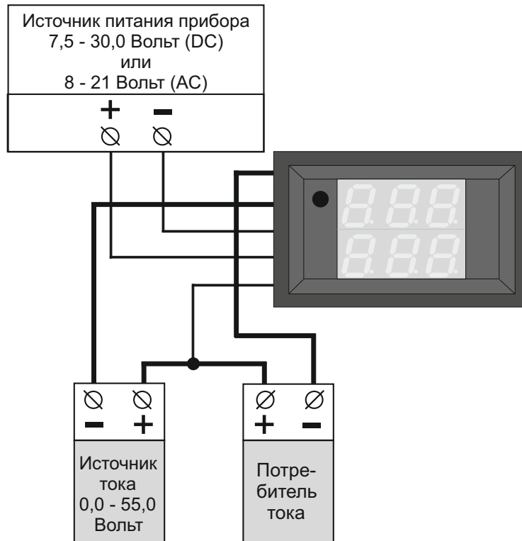
Рис. 4. Вариант измерения напряжения и потребляемого тока от источника с выходным напряжением от 0,00 до 55,0V.
