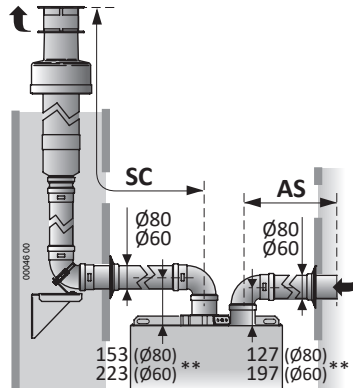
Приклад роздільної системи (C 53 )
