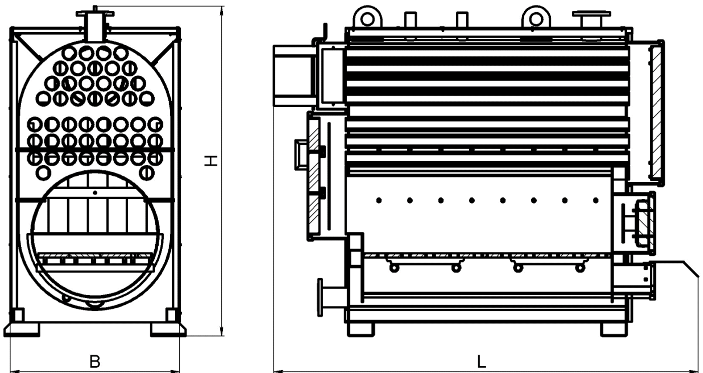
Рисунок 3.1 – Позначення габаритів котла типу КТУ (потужністю 99-600 кВт)
