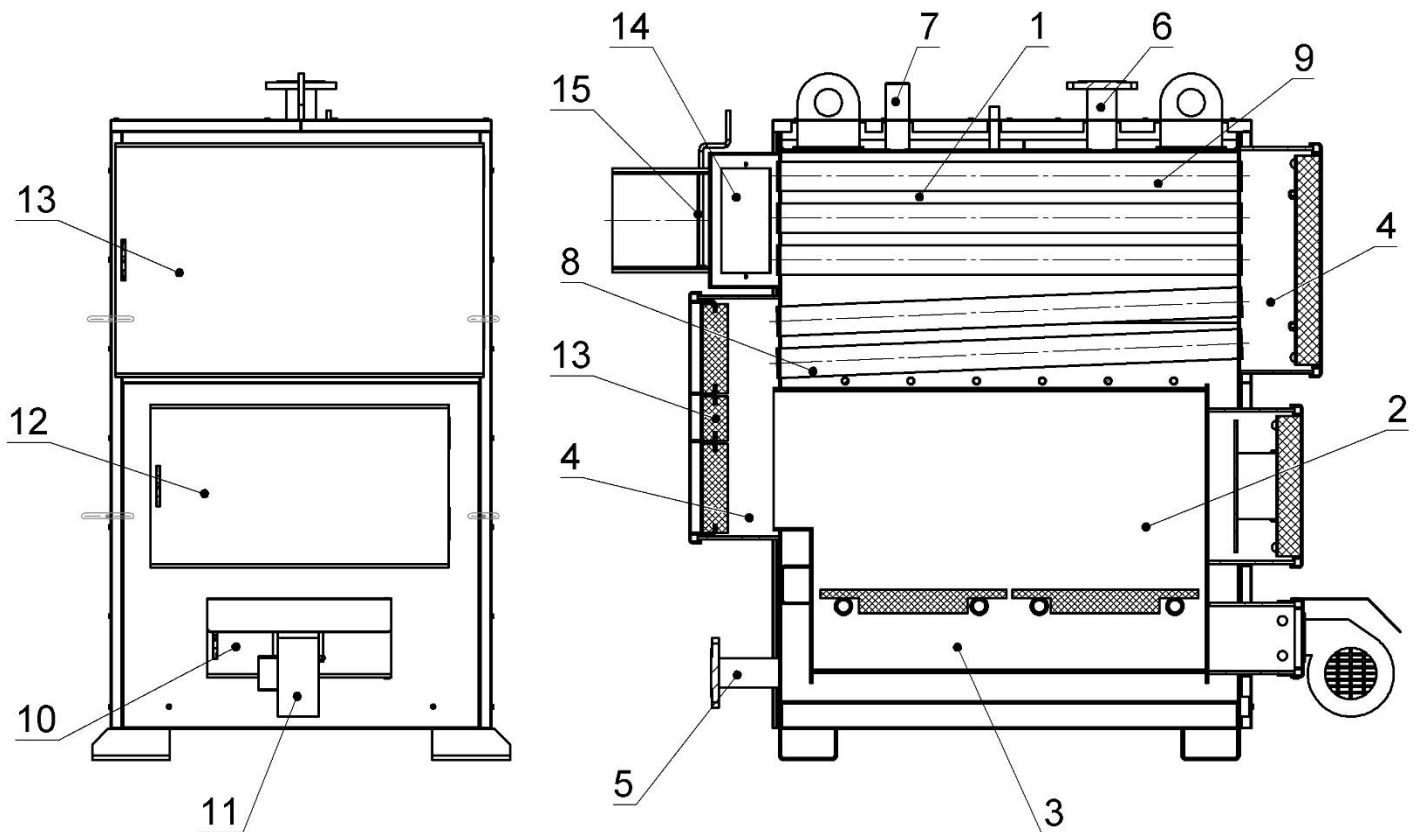
Рисунок 5.1 – Зовнішній вигляд та основні елементи котла типу КТУ
