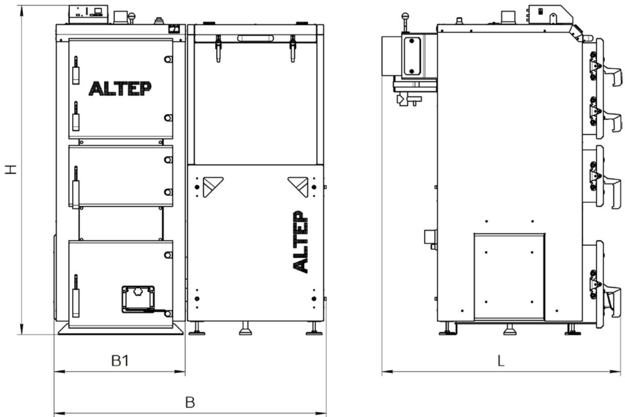
Рисунок 1 – Габаритне креслення котла типу КТ-2Е-ШН
