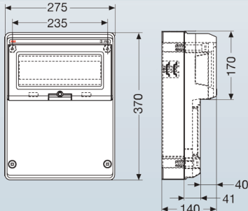
Размеры щита автоматики TRK
