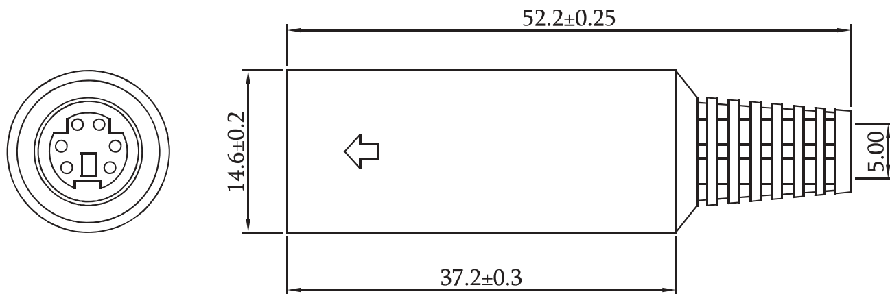
Размеры, мм
