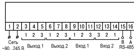
Рисунок 5.2 – Назначение контактов клеммника ТРМ202-Н, -Щ1 и -Щ2
