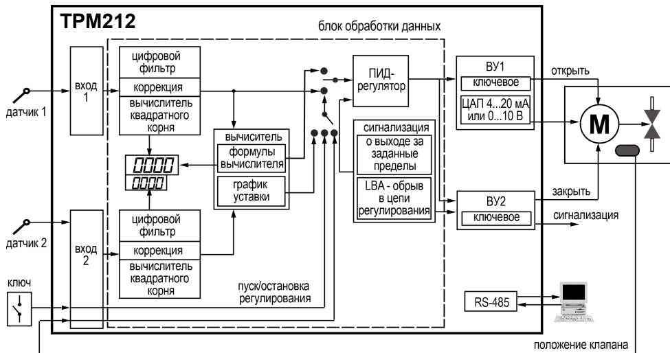
Рисунок 6.1 – Функциональная схема прибора
