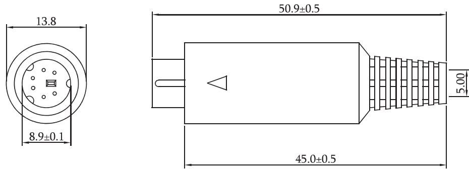
Размеры, мм
