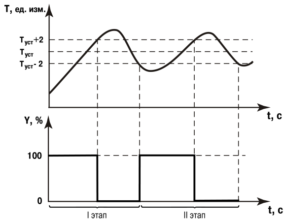
Рисунок 7.14 – АНР прибора, работающего в режиме нагревателя
