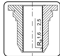
Растачивание отверстий
