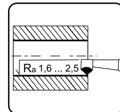
Растачивание отверстий
