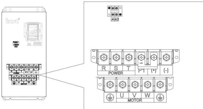
Рис.4-14. 75~110 кВt клеммы силовых цепей
