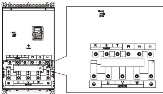
Рис.4-15. 132~200 кВt клеммы силовых цепей
