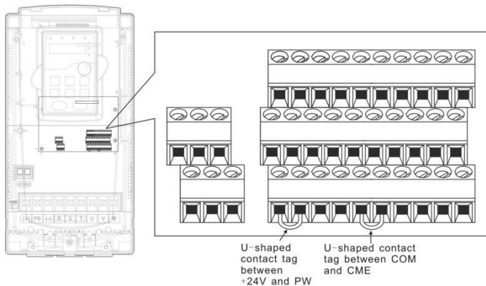
Рис. 4-21. U-образный контакт
