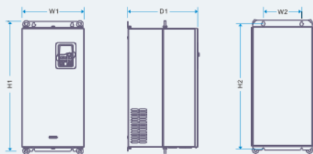
Схема установки для ПЧ 18—55кВт
