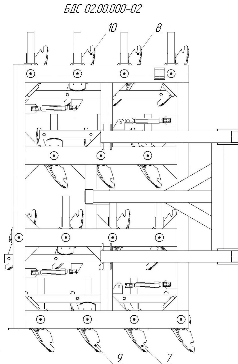
Рис. 9 Крыло левое в сборе БДС 02.00.000-01(-02) для бороны дисковой модульной прицепной ANTARES 6x4C (выпускается с 2016 г.)
