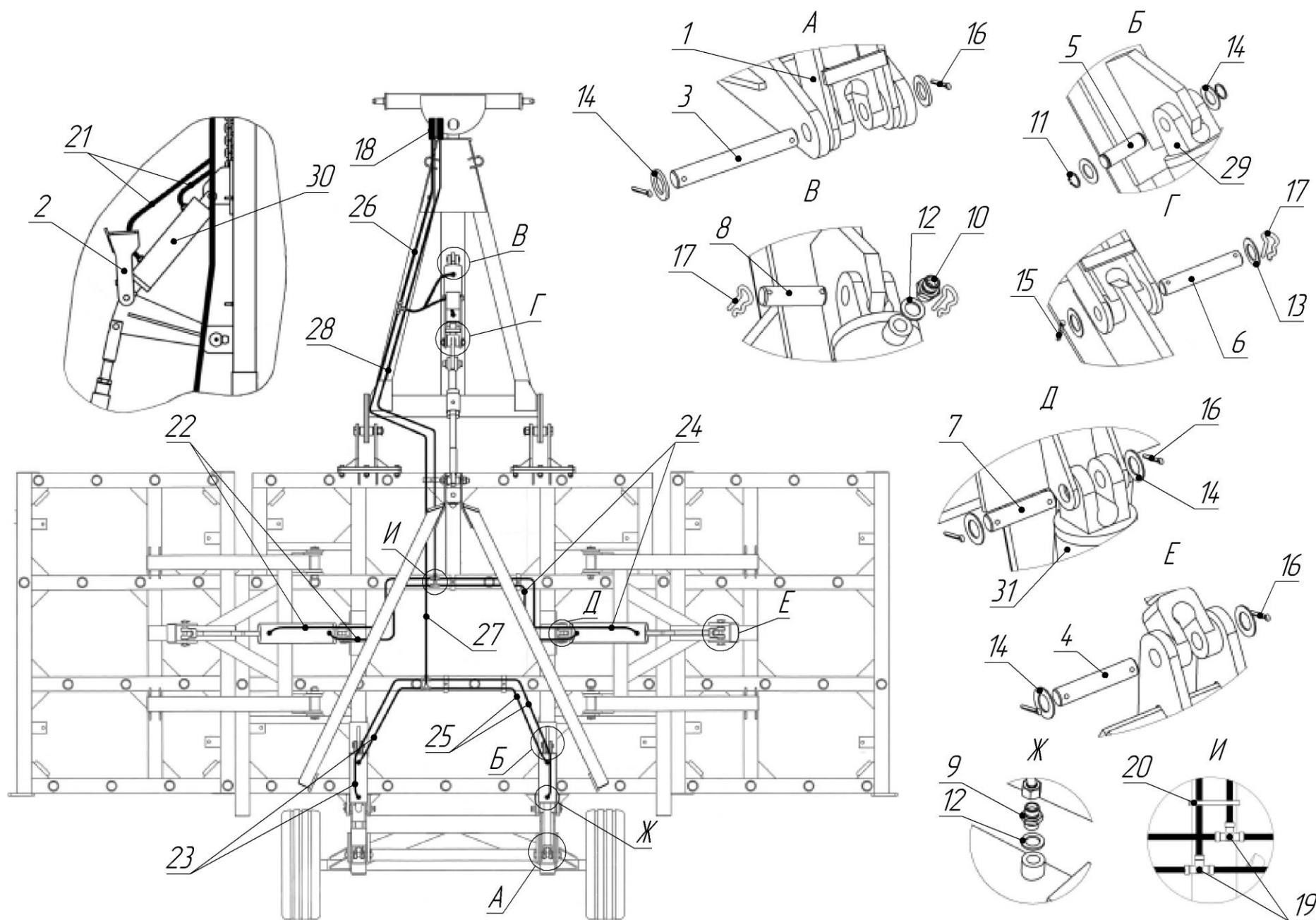
Рис. 27 Гидротрасса БДС 25.00.000-01 для борны дисковой модульной прицепной ANTARES 6x4C
