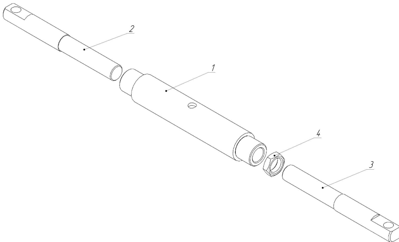
Рис. 22 Талреп БДУ 26.00.000 для бороны дисковой модульной прицепной ANTARES 6x4C (выпускается с 2016 г.)
