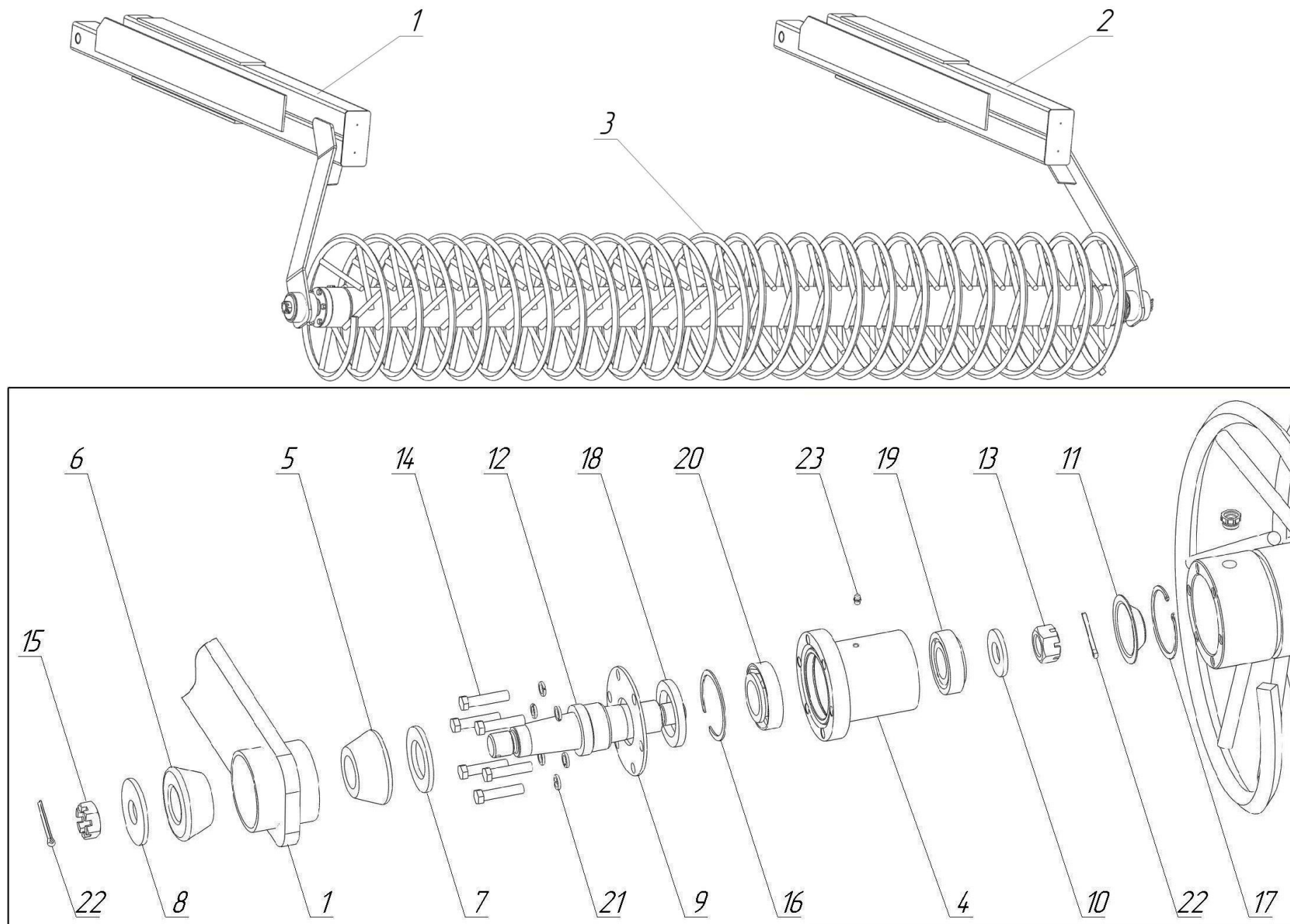
Рис. 17 Шлейф-каток БДС 10.00.000 для бороны дисковой модульной прицепной ANTARES 6x4С
