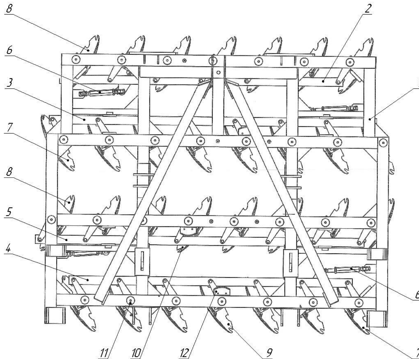
Рис. 4 Рама в сборе БДС 01.00.000 для борны дисковой модульной прицепной ANTARES 6x4С (выпущена до 2016 г.)
