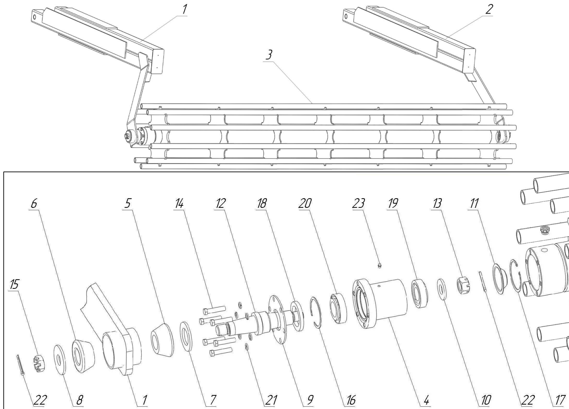
Рис. 18 Каток БДС 10.00.000-01 для бороны дисковой модульной прицепной ANTARES 6x4C
