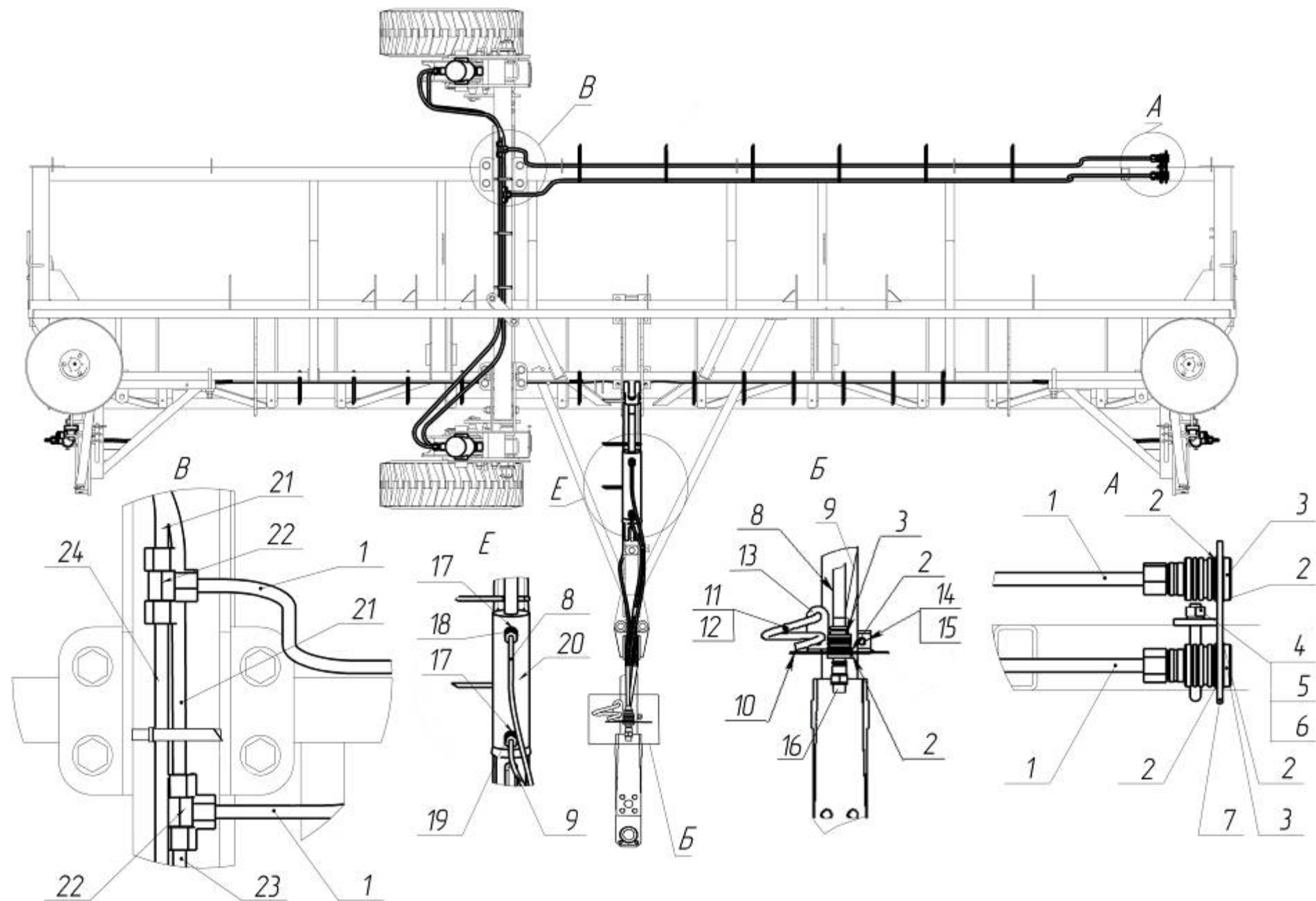
Рис. 18 Гидротрасса.
