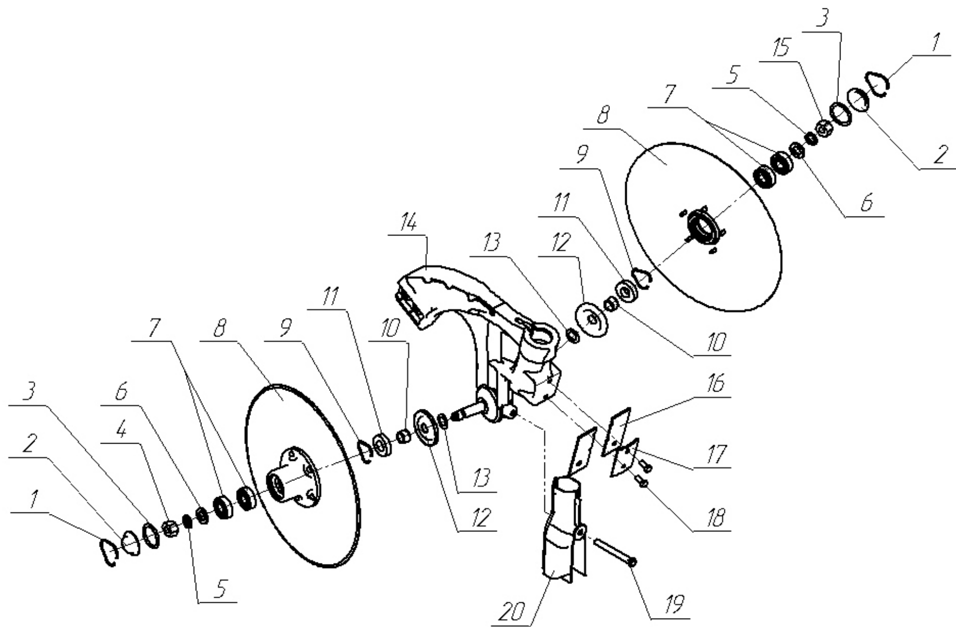
Рис. 12 Сошник Н 105.04.000.
