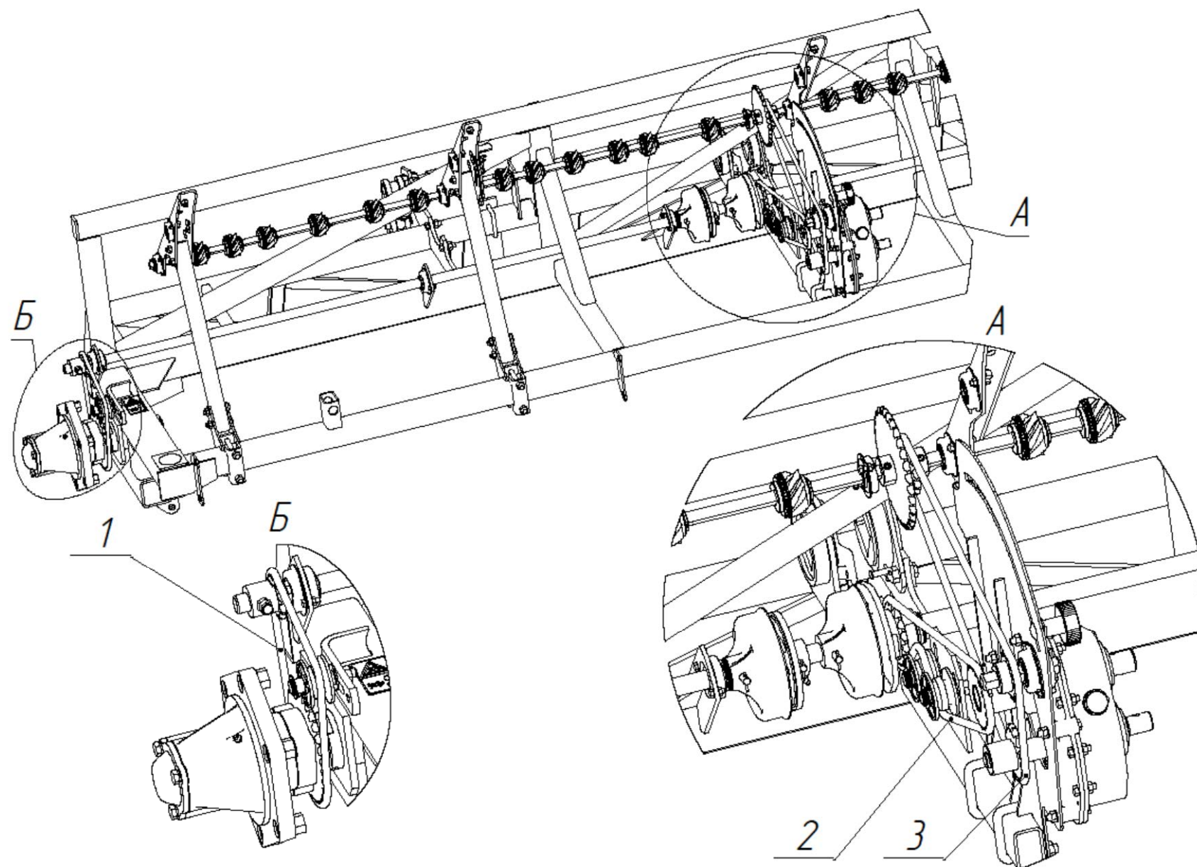
Рис. 8 Механизм привода зерновых высевающих аппаратов.
