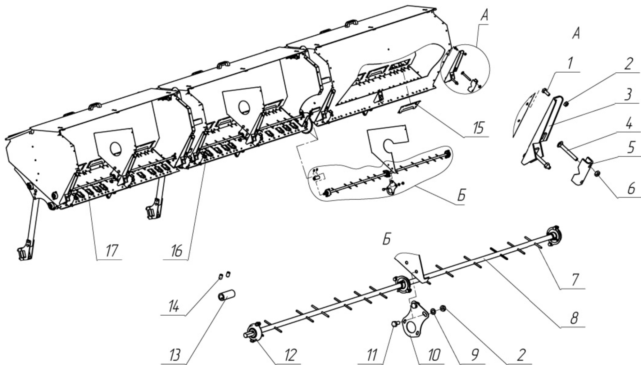
Рис. 3.5 Валы ворошилок
