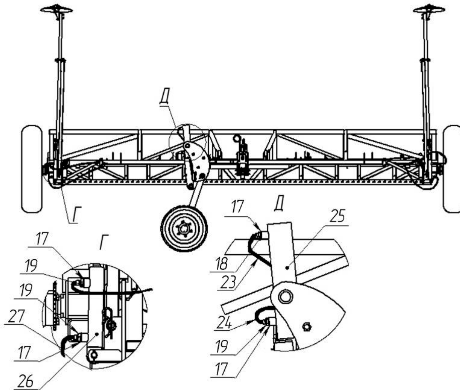
Рис. 18.1 Гидротрасса (продолжение).
