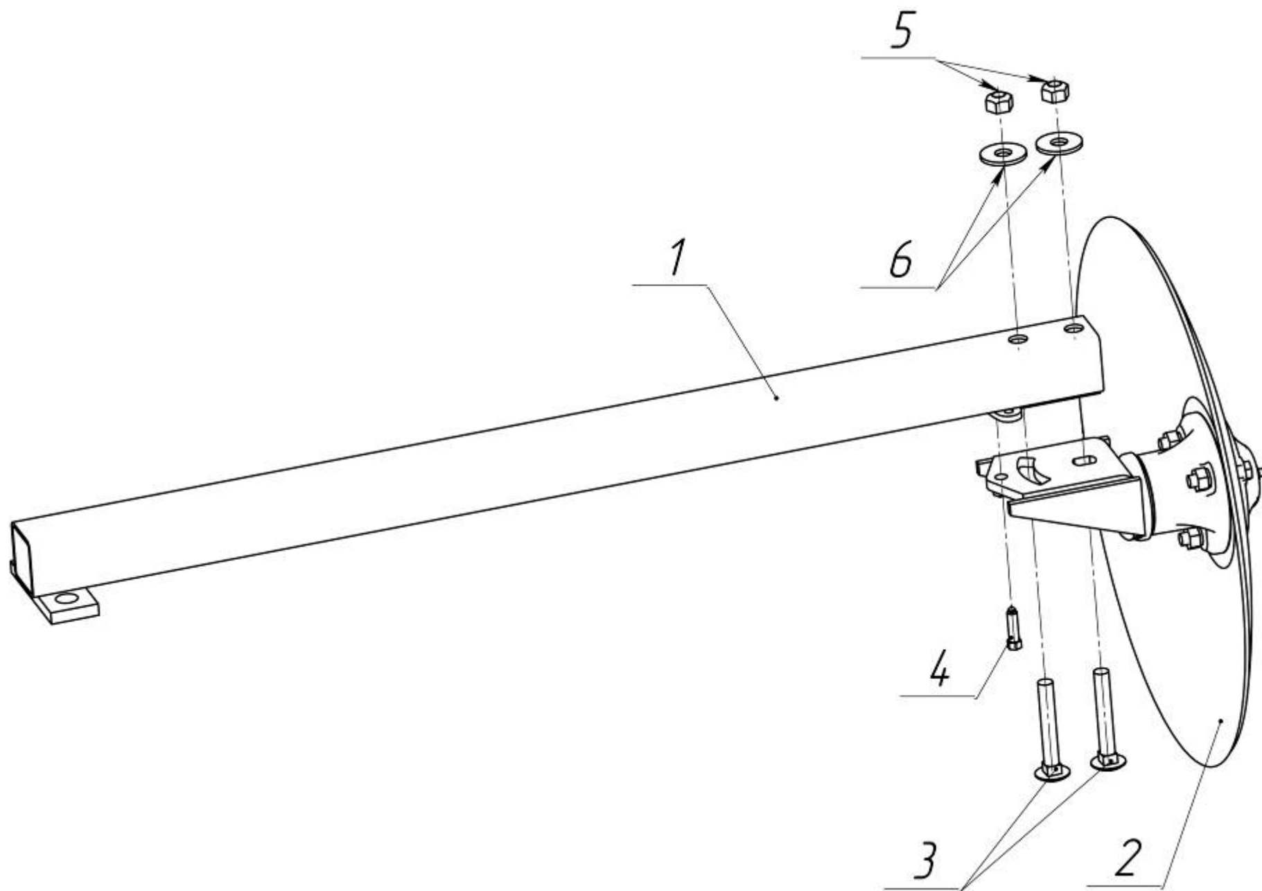
Рис. 16.1 Удлинитель ОЗШ 01.540.
