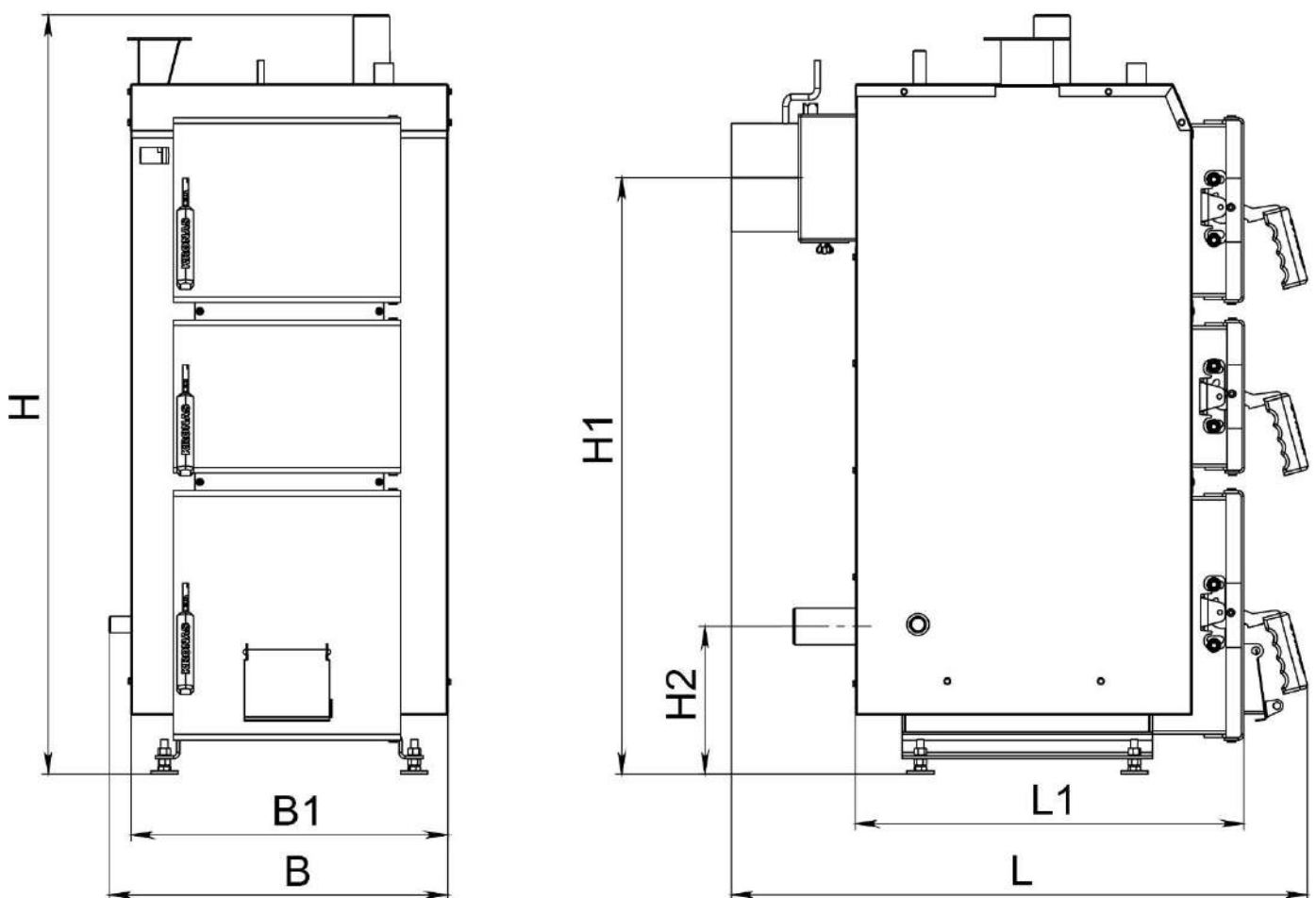
Рисунок 3.1 – Позначення габаритів котла типу К (потужністю 15-30 кВт)
