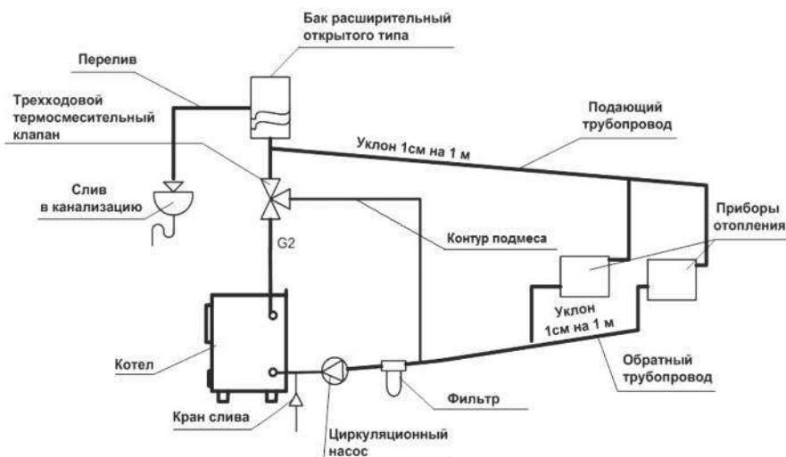
Рис.3 Схема открытой системы водяного отопления
