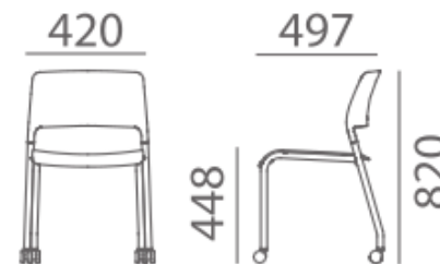
Габаритные размеры
