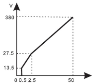
Кривая с постоянным крутящим моментом
