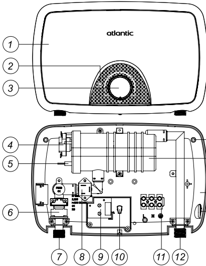
МОДЕЛЬ: Ivory IV202, Ivory IV202 SB (5.5 kW)
