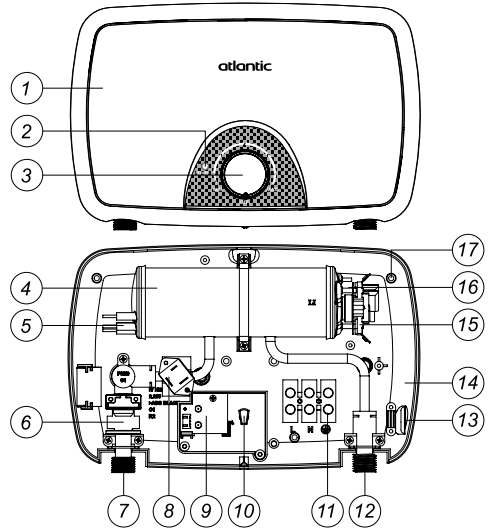
МОДЕЛЬ: Ivory IV202, Ivory IV202 SB (7 kW)
