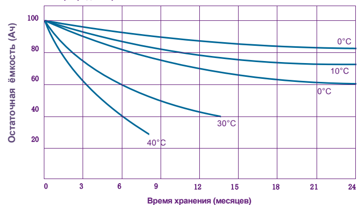
Саморазряд батарей
