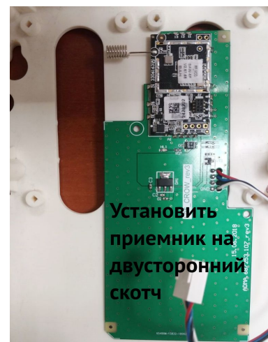
Рисунок 27. Адаптер «L25_Crow_rev3» в корпусе прибора
