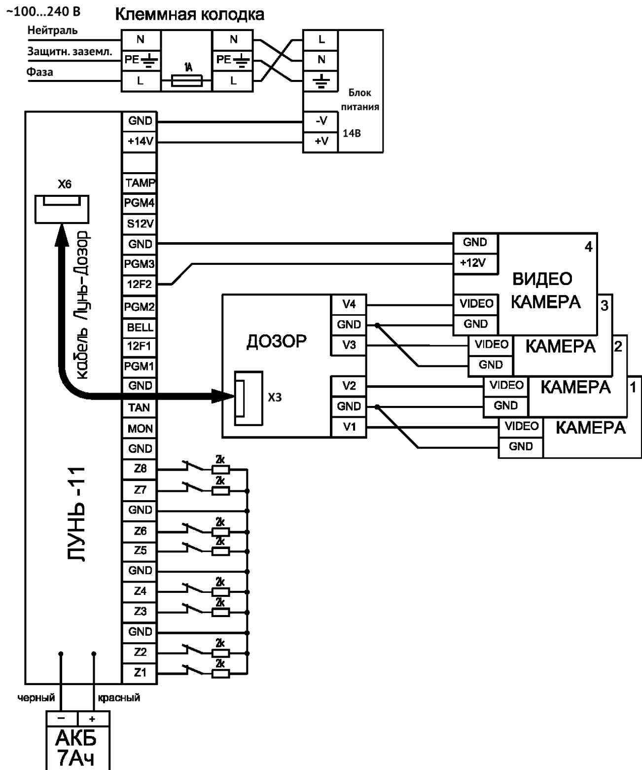
Рисунок 42. Схема подключения модуля фотоподтверждения тревог «Дозор»
