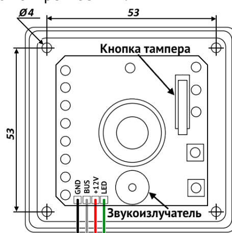
Рисунок 11. УИУ «Линд-11ТМ» без крышки
