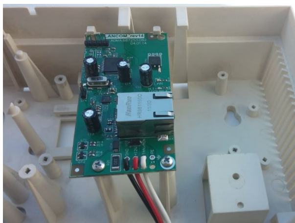
Рисунок 31. Коммуникатор «LanCom11» rev.14 в корпусе прибора
