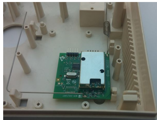
Рисунок 22. Радиоприемник «MCR-300» Visonic в корпусе прибора
