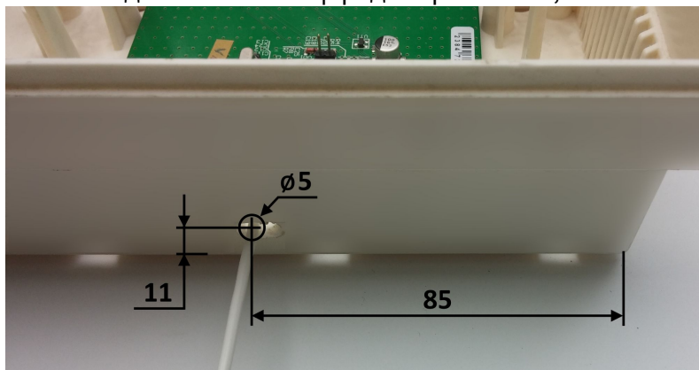
Рисунок 21. Отверстие в корпусе для антенны радиоприемника «P433» rev.4
