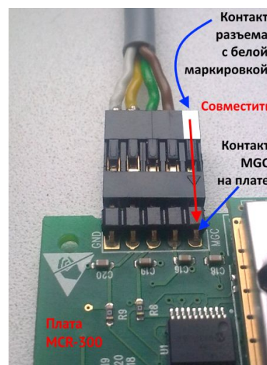
Рисунок 23. Подключение радиоприемника Visonic
