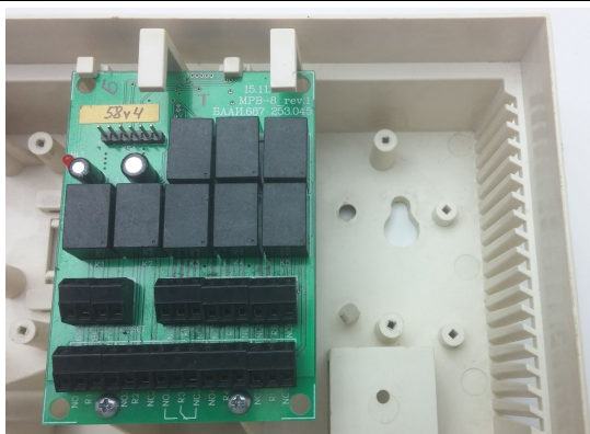
Рисунок 18. Модуль «МРВ-8М» в корпусе прибора
