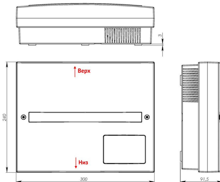
Рисунок 2. Габаритные размеры корпуса ППКОП
