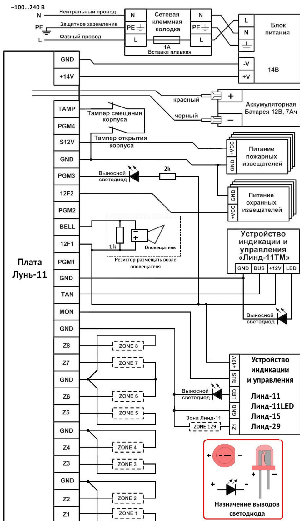
Рисунок 39. Схема подключения ППКОП
