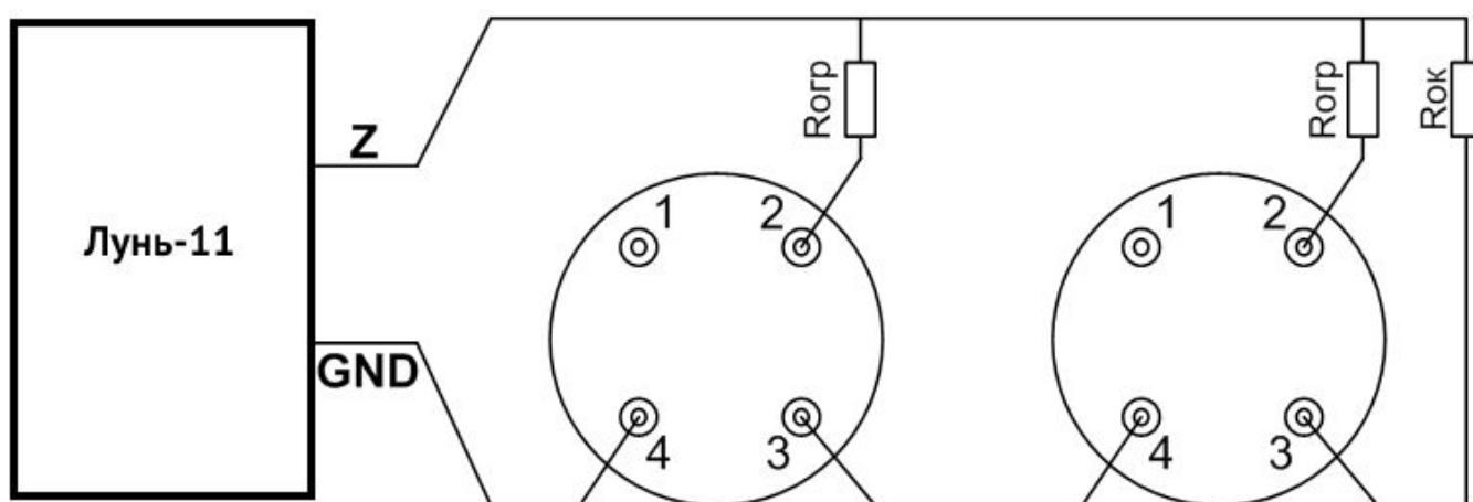
Рисунок 38. Схема подключения извещателей в пожарный шлейф по двухпроводной схеме
