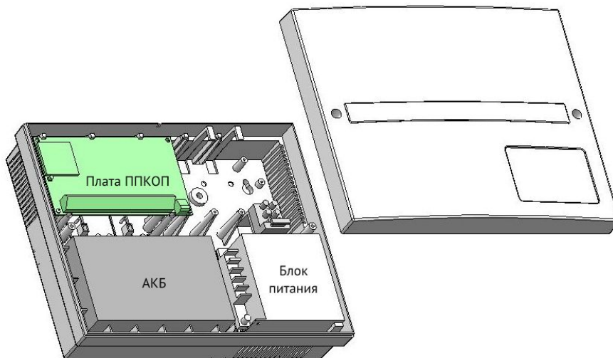
Рисунок 1. Размещение компонентов ППКОП в корпусе
