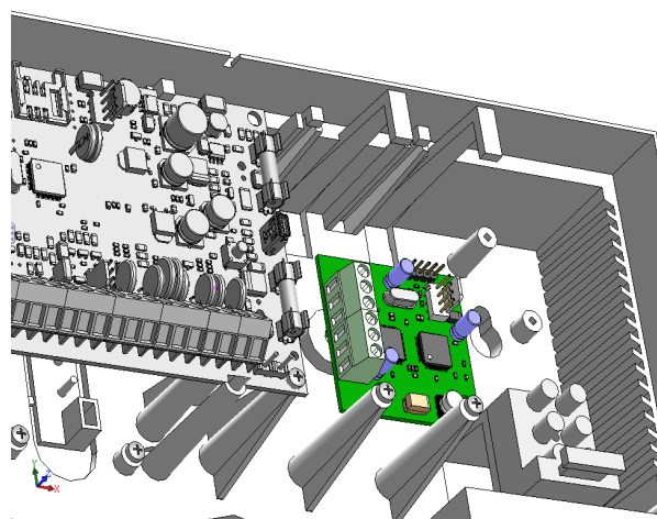
Рисунок 33. Установка модуля «Дозор»
