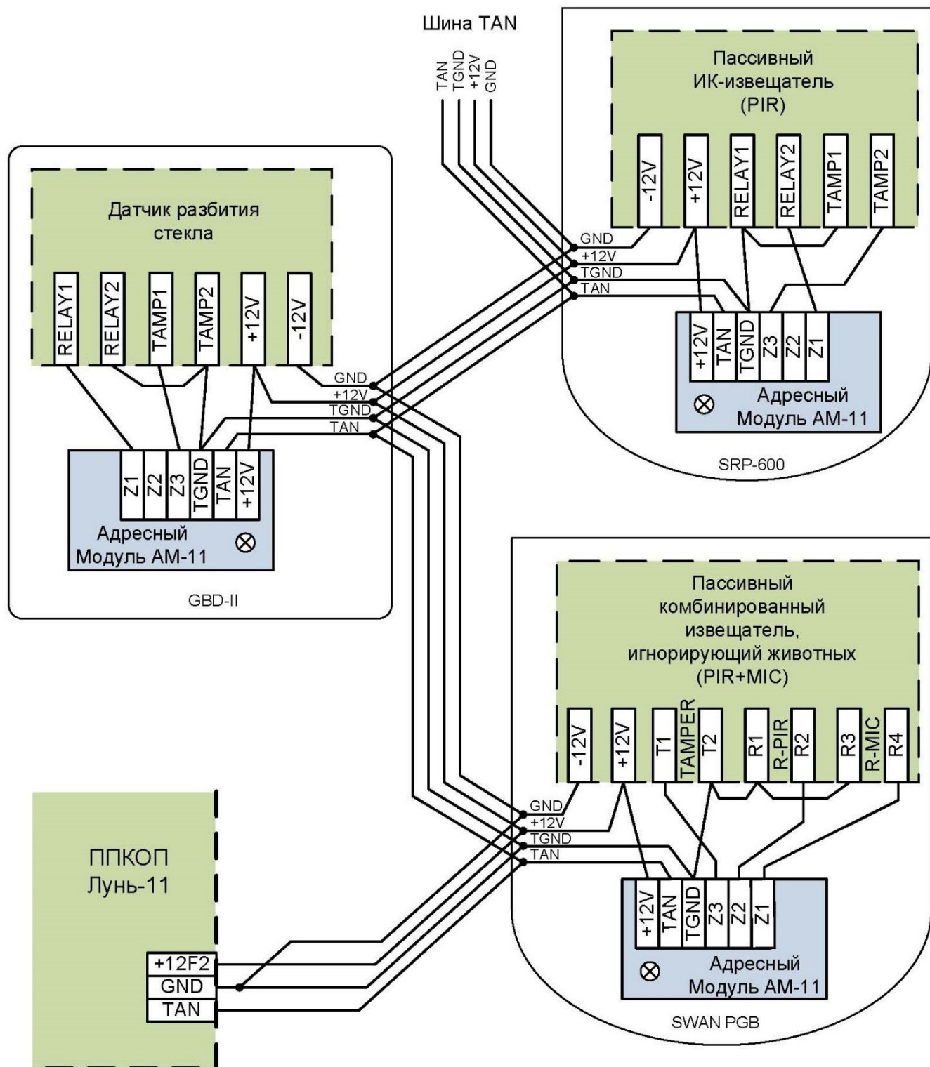
Рисунок 40. Пример использования адресных модулей «АМ-11»
