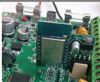
Рисунок 35. Установка модуля «W11M» в X3
