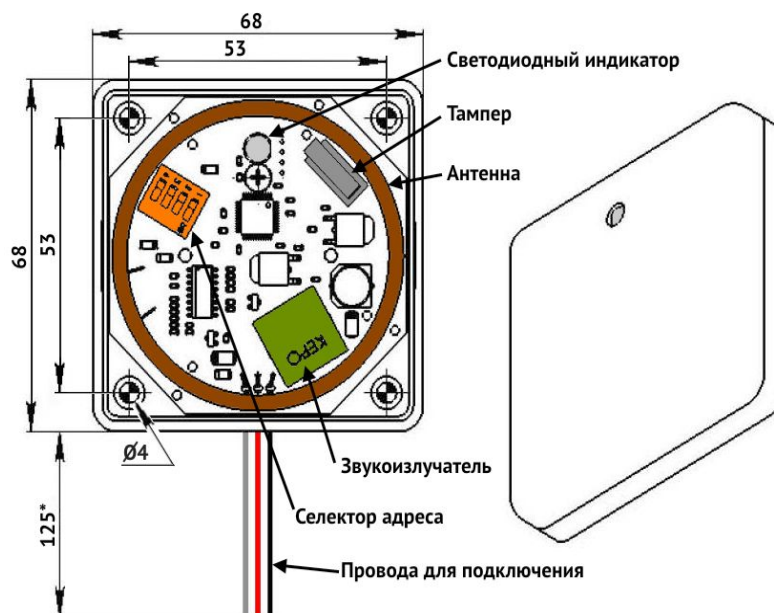
Рисунок 12. Внешний вид и устройство УИУ «Линд-ЕМ»
