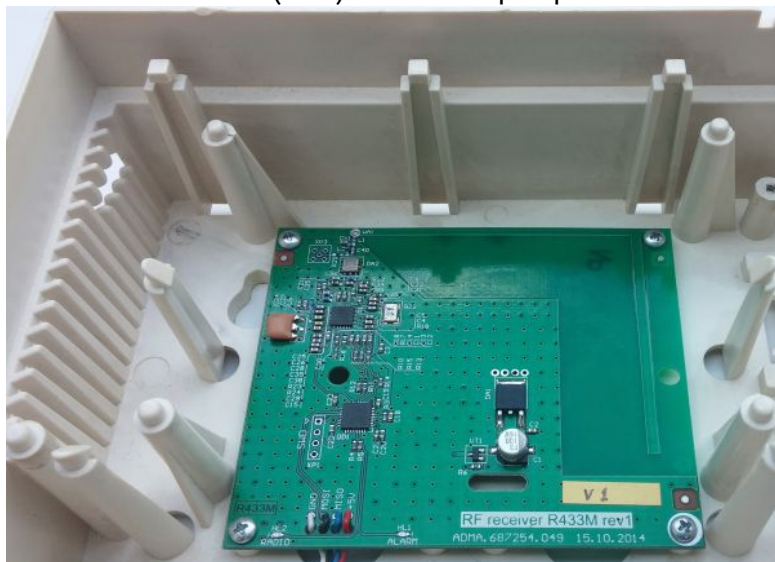
Рисунок 19. Радиоприемники серии «P433» в корпусе прибора
