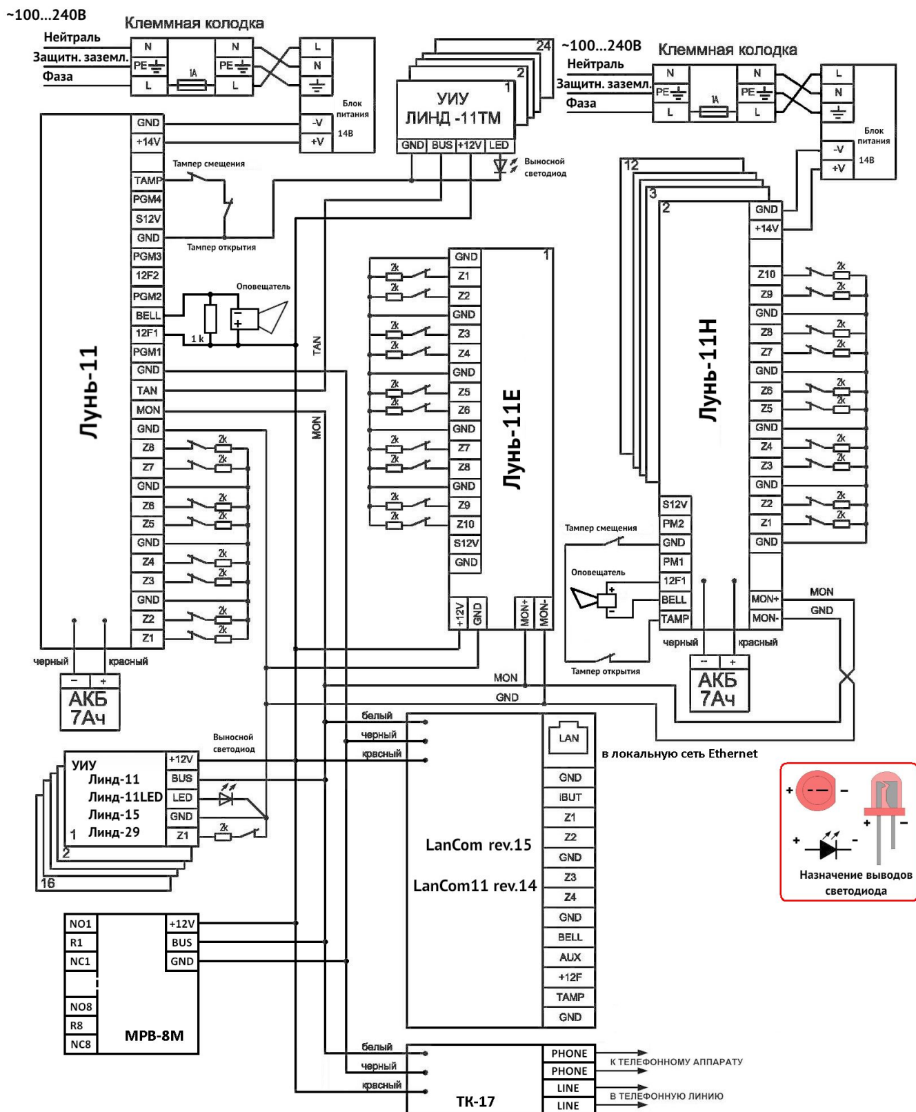
Рисунок 41. Схема подключения сетевых устройств
