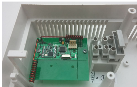
Рисунок 29. Радиоприемник Ajax «uartBridge» в корпусе прибора
