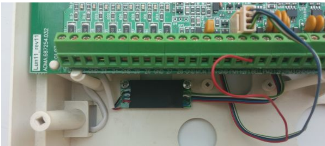
Рисунок 24. Установка и подключение адаптера «Астра-Лунь11»
