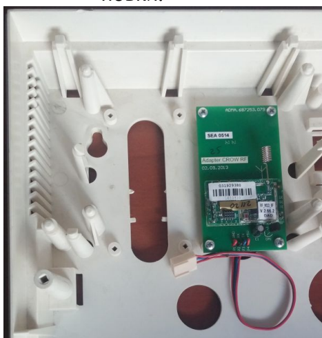
Рисунок 25. Адаптер «Crow – Лунь- 11» в корпусе прибора
