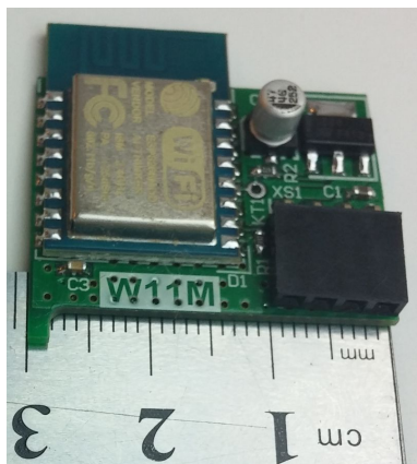
Рисунок 34. Общий вид модуля «W11M»
