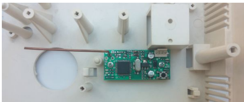
Рисунок 28. Радиоприемник Ajax «RR-108» в корпусе прибора
