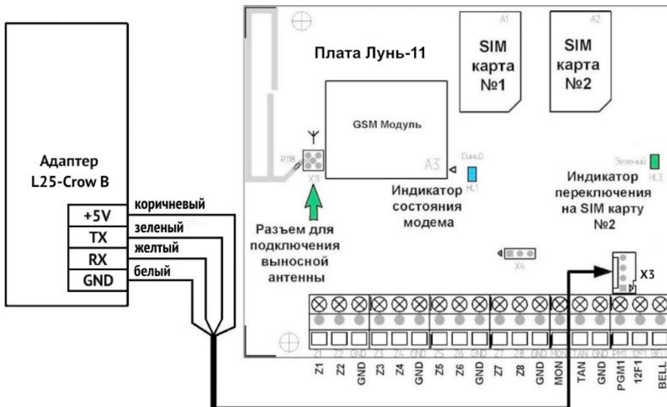
Рисунок 45. Схема подключения адаптера «L25-Crow B»
