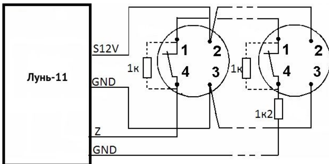
Рисунок 37. Схема подключения пожарных извещателей по четырехпроводной схеме
