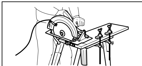
O ilustrare tipică de sprijinire corectă a mâinii, sprijinire a piesei și amplasare a cablului de alimentare (dacă este cazul).
