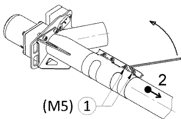
Рис.4 Демонтаж трубы шнека
