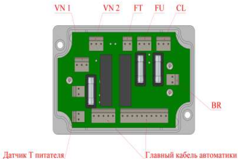
Рис.4 Схема подключений в блоке коммутации горелки KVIT Optima R
