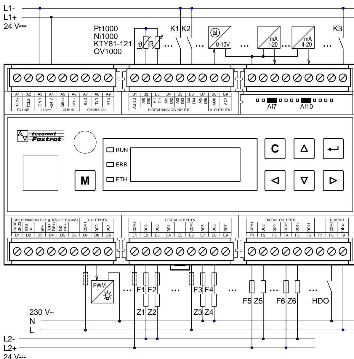
Obr. 4.1 Příklad zapojení binárních a analogových vstupů/výstupů základního modulu CP-1016
