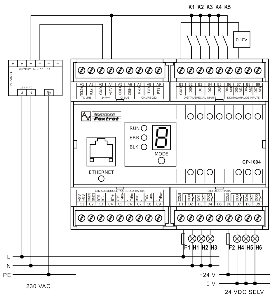
Obr. 4.1 Základní zapojení modulu CP-1004
