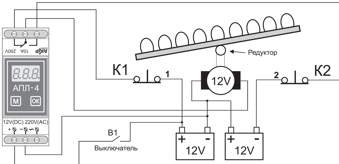
Рис. 2. Вариант схемы подключения с реверсом и питанием от 12 Вольт.
