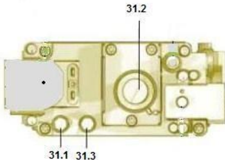
Рис. 6.3-1 Детали газового блока HNB-120
