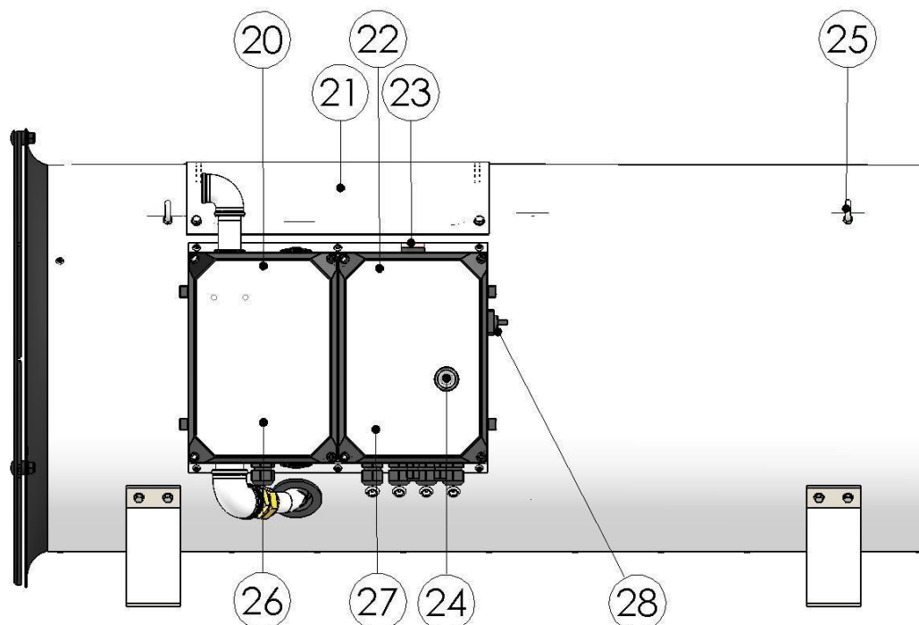
Рис.6.2-1 Пульт управления – вид спереди
