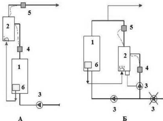
Рис. 4 – Комбинированное отопление. Схемы подключения электрокотла
