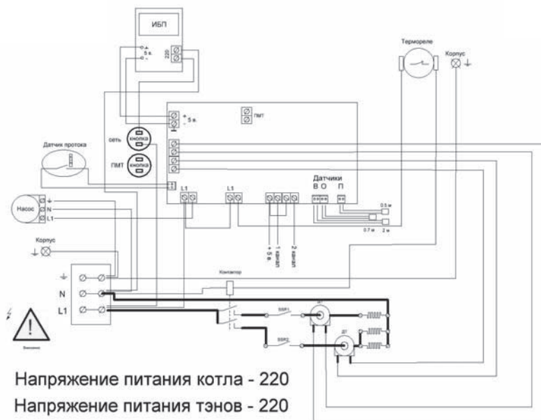
Схема электрическая котла "Премиум"
