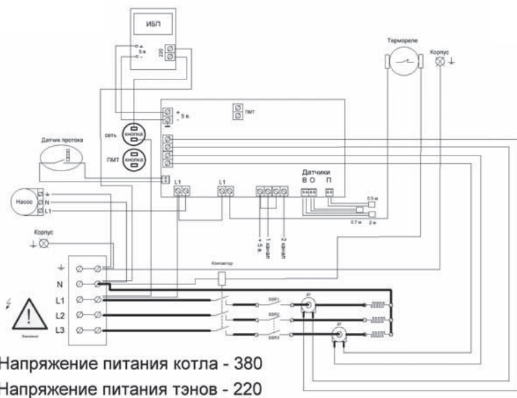
Схема электрическая котла "Премиум"
