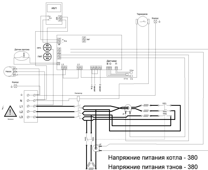
Схема электрическая котла "Премиум Плюс"
