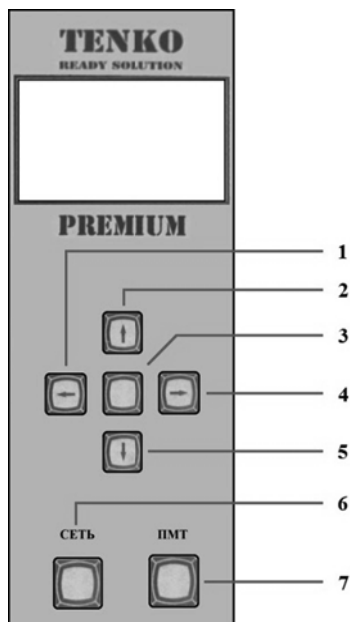
Рис. 5 – Лицевая панель котла
